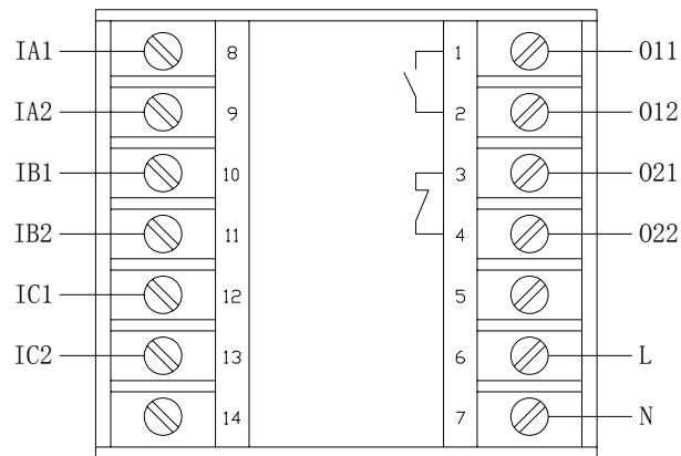
AMDTH-X/F004 系列主单元端子图
