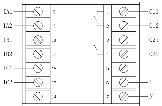
AMDTH-X/F003 系列主单元端子图
