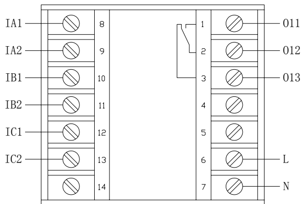
AMDTH-X/F001 系列主单元端子图
