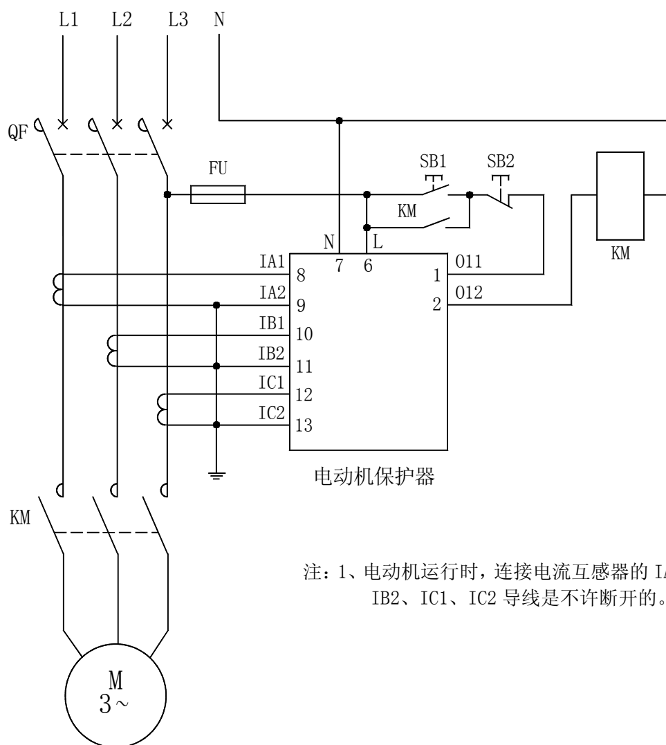
AMDTH-X/F00□ 系列电动机保护器应用电气原理图
