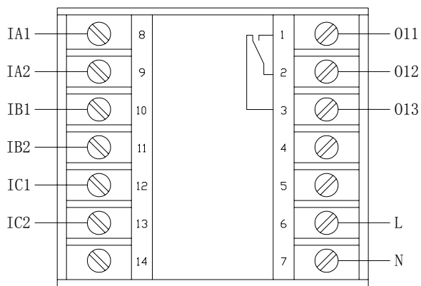
AMDTH-X/E021 主单元端子图
