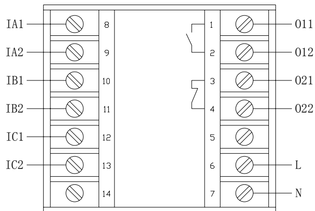
AMDTH-X/E024 主单元端子图
