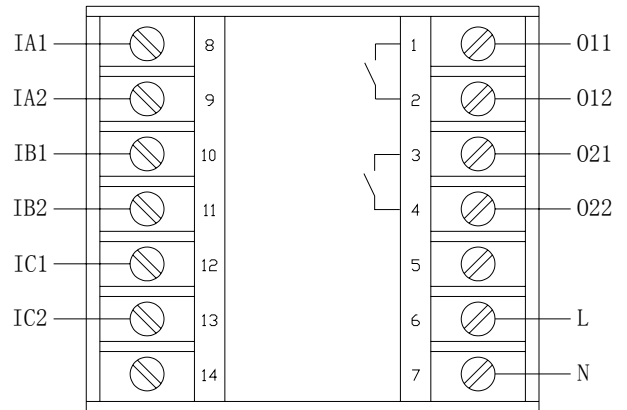
AMDTH-X/E023 主单元端子图
