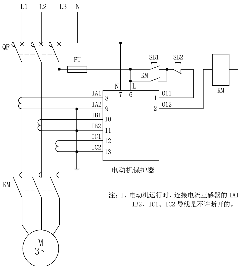
AMDTH-X/E02□ 系列电动机保护器应用电气原理图
