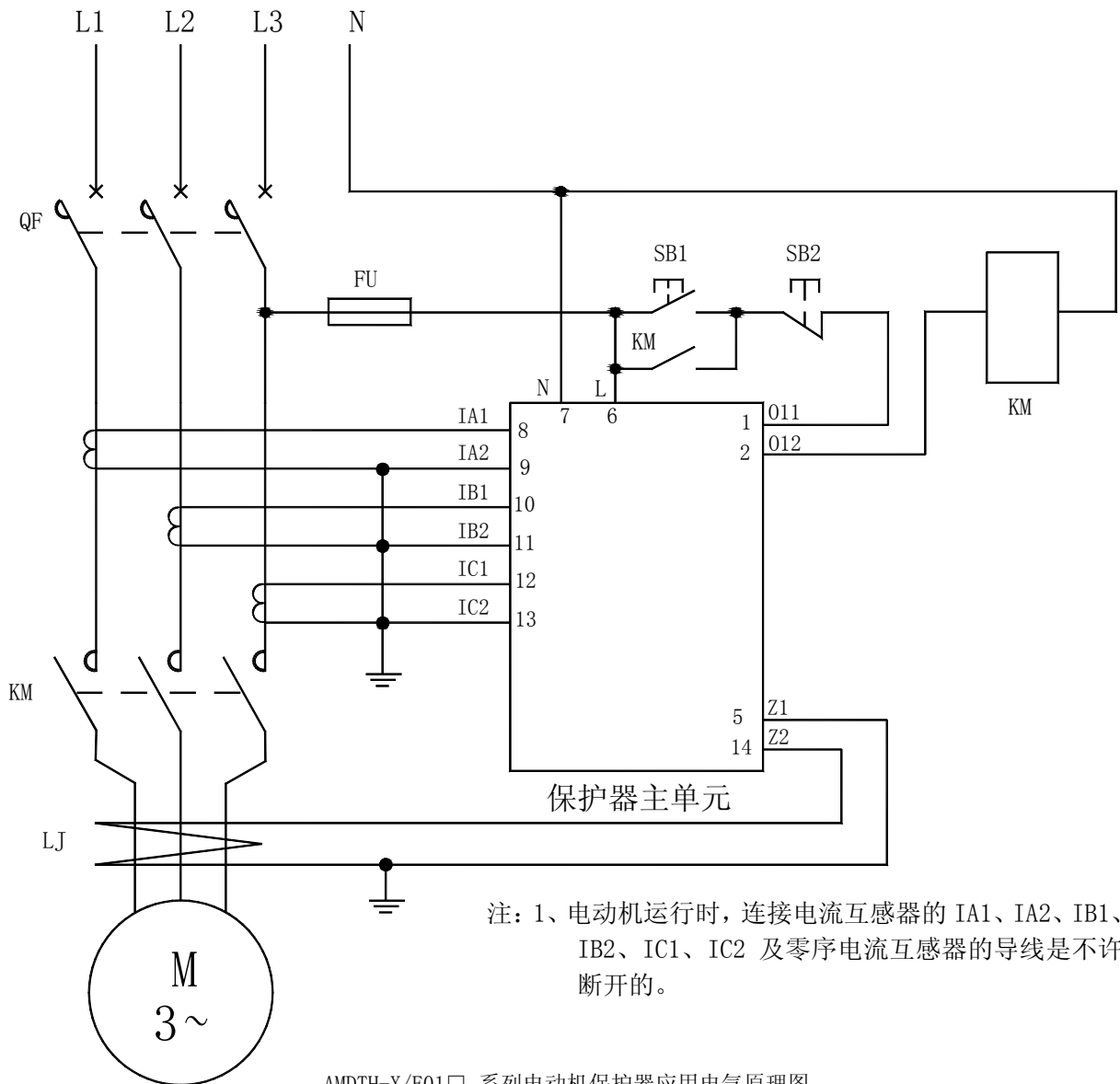
AMDTH-X/E01□ 系列电动机保护器应用电气原理图
