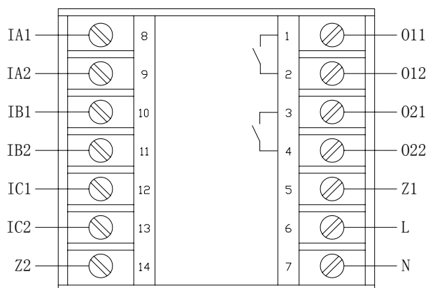
AMDTH-X/E013 主单元端子图
