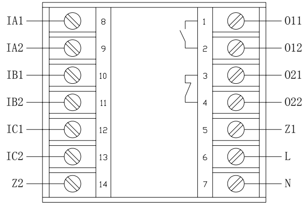
AMDTH-X/E014 主单元端子图
