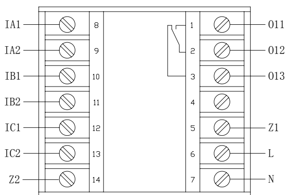
AMDTH-X/E011 主单元端子图
