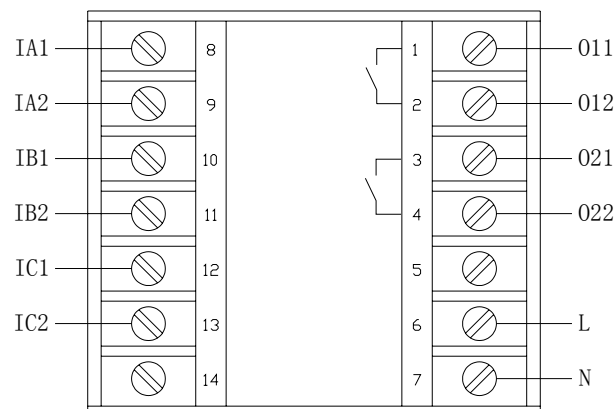
AMDT-X/F043 系列主单元端子图
