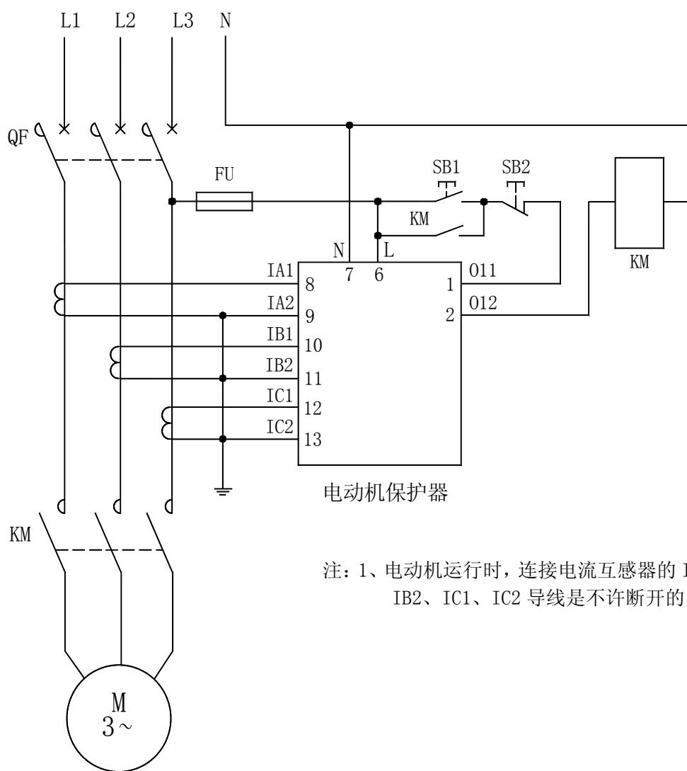
AMDT-X/F04□ 系列电动机保护器应用电气原理图
