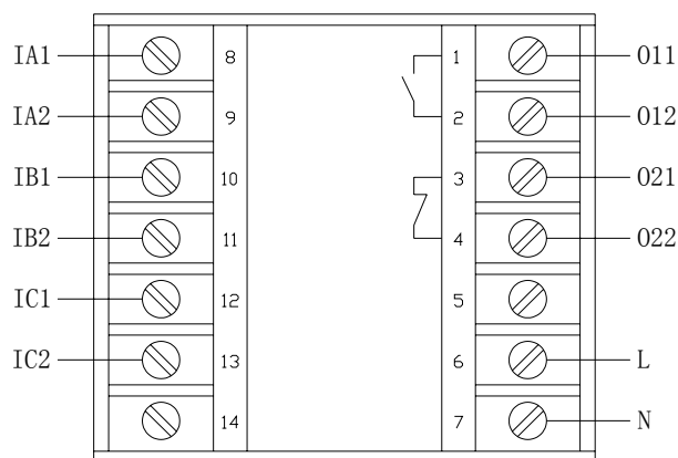
AMDT-X/F044 系列主单元端子图
