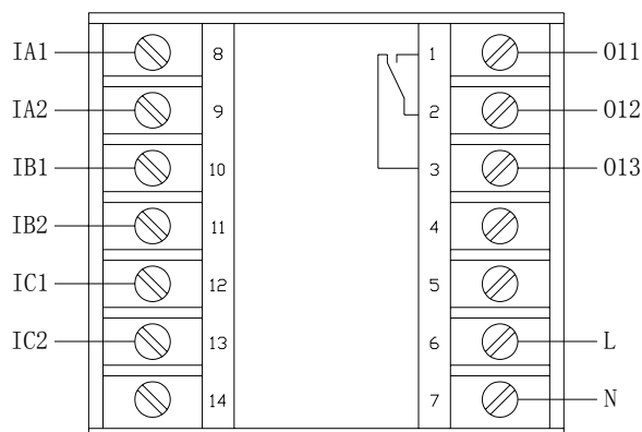
AMDT-X/F041 系列主单元端子图
