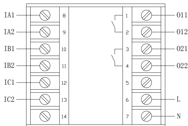
AMDT-X/F033 系列主单元端子图
