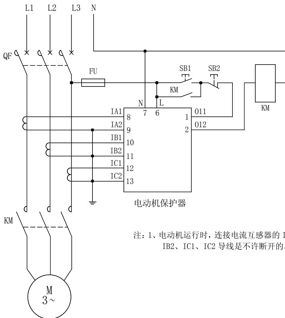
AMDT-X/F03□ 系列电动机保护器应用电气原理图
