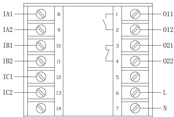
AMDT-X/F034 系列主单元端子图
