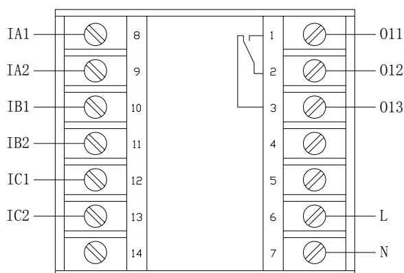
AMDT-X/F031 系列主单元端子图
