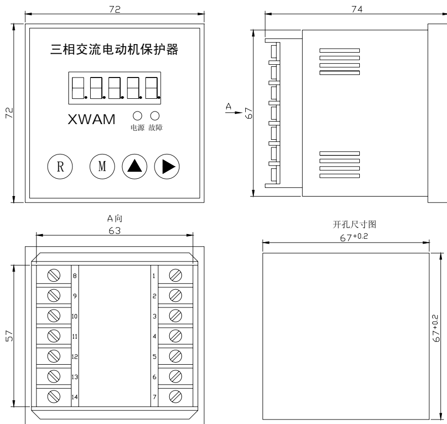
AMDT-X/F03□ 系列电动机保护器主单元外形及安装孔尺寸
