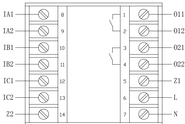
AMDT-X/E053 主单元端子图
