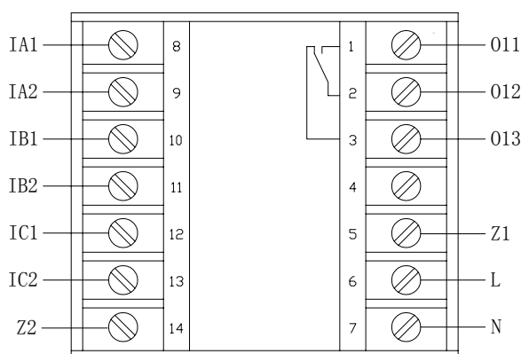
AMDT-X/E051 主单元端子图
