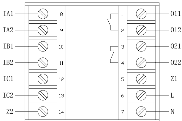
AMDT-X/E054 主单元端子图
