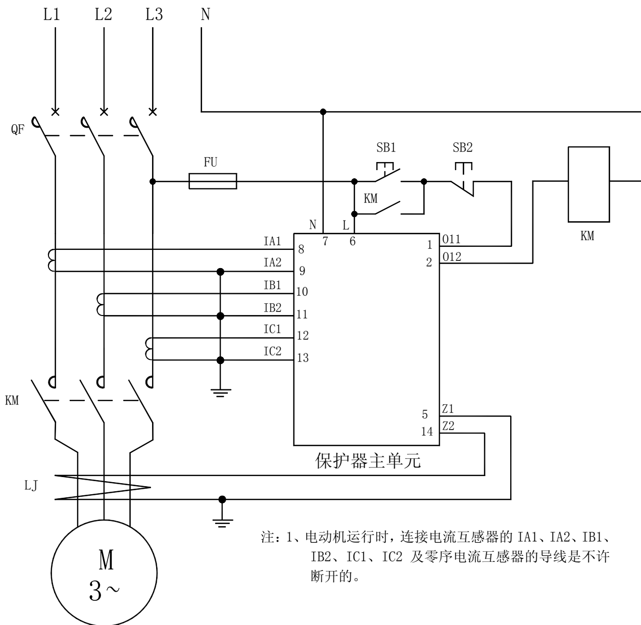
AMDT-X/E054 系列电动机保护器应用电气原理图
