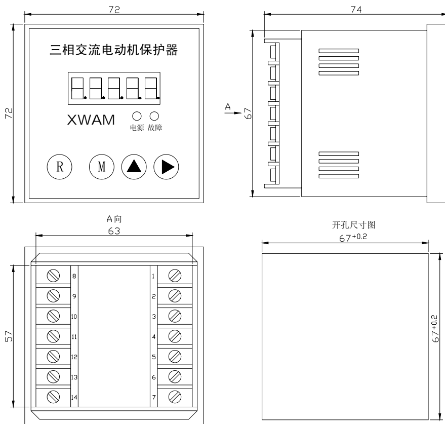
AMDT-X/E05□ 系列电动机保护器主单元外形及安装孔尺寸
