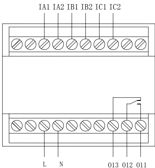
AMDSH-X/E021 主单元端子图
