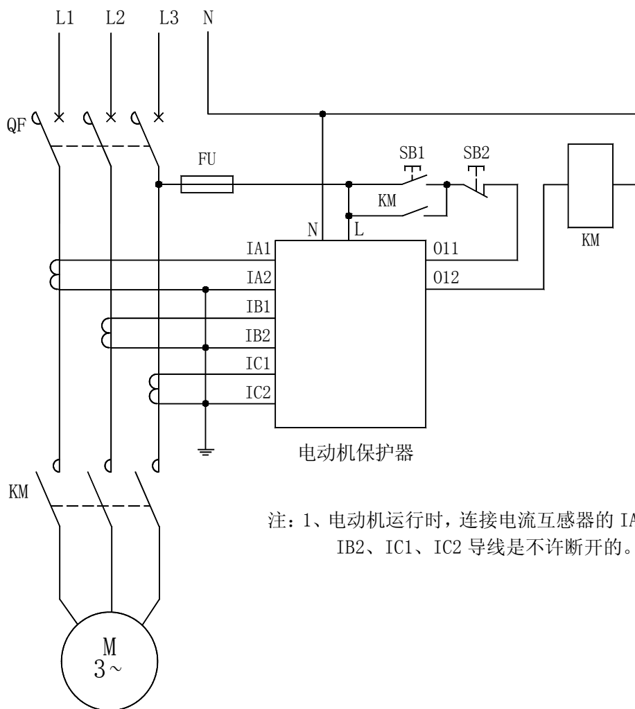
AMDSH-X/E02□ 系列电动机保护器应用电气原理图
