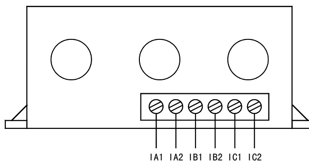
AMDSH-□/DO3□ 系列保护器电流检测单元接线端子图
