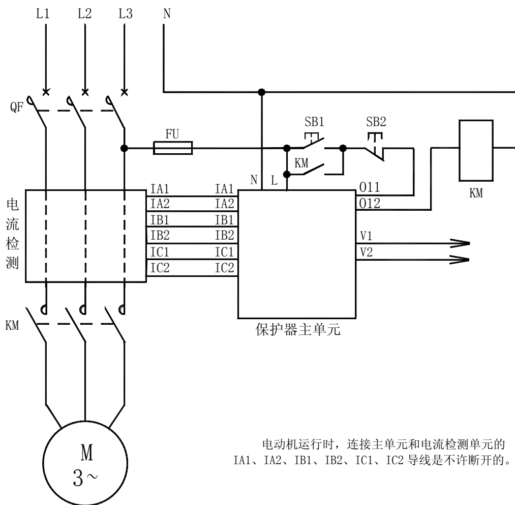
AMDSH-□/DO3□ 系列电动机保护器应用电气原理图
