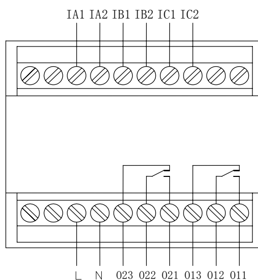
AMDSH-□/DO32 系列保护器主单元接线端子图
