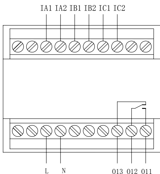
AMDSH-□/DO31 系列保护器主单元接线端子图
