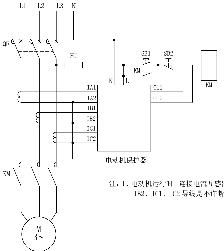
AMDS-X/F04□ 系列电动机保护器应用电气原理图
