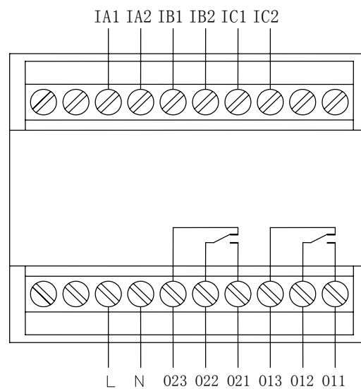
AMDS-X/F042 主单元端子图
