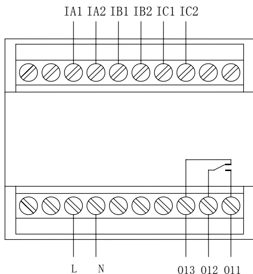
AMDS-X/F041 主单元端子图
