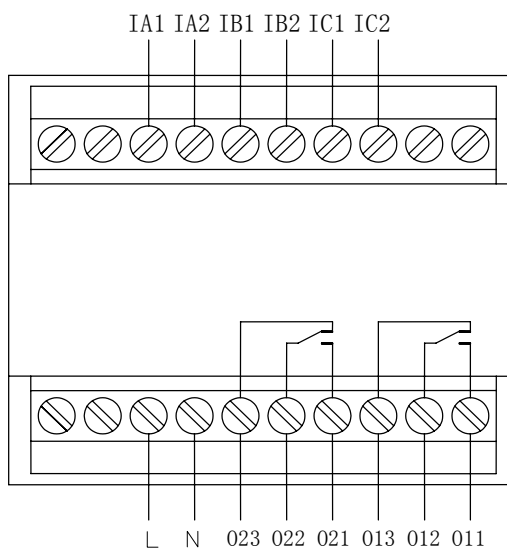
AMDS-X/F032 主单元端子图
