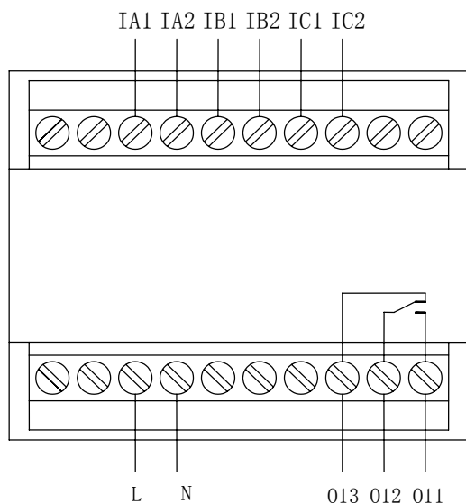
AMDS-X/F031 主单元端子图
