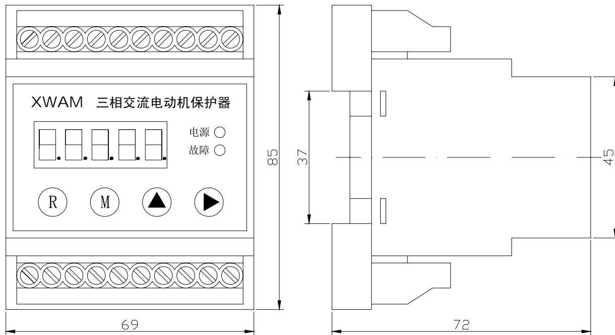
AMDS-X/F03□ 系列电动机保护器主单元外形及安装孔尺寸
