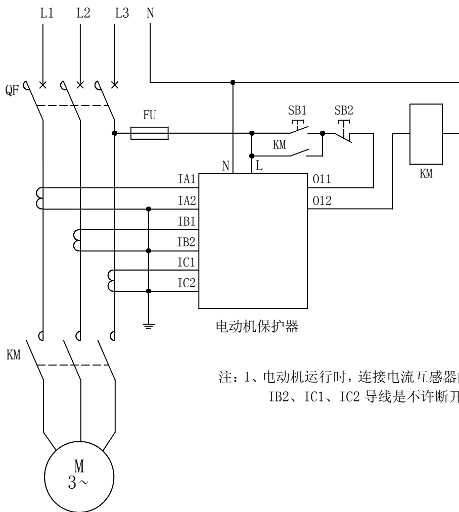
AMDS-X/F03□ 系列电动机保护器应用电气原理图
