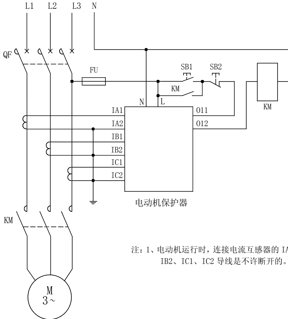
AMDS-X/F02□ 系列电动机保护器应用电气原理图
