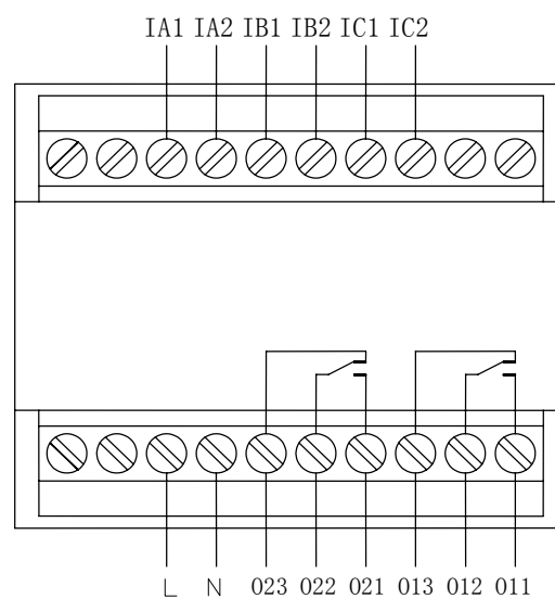
AMDS-X/F022 主单元端子图
