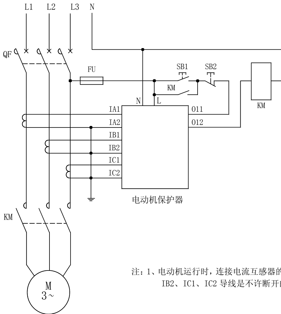
AMDS-X/F00□ 系列电动机保护器应用电气原理图
