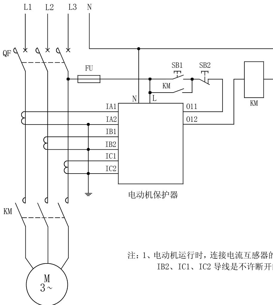
AMDS-X/E02□ 系列电动机保护器应用电气原理图
