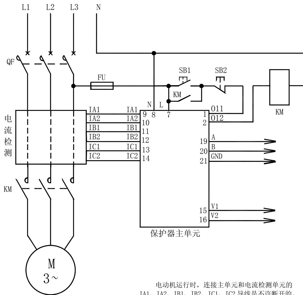
AMDP-□/□D24□ 系列电动机保护器应用电气原理图
