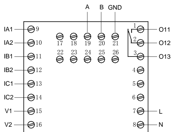
AMDP-□/□D241 系列保护器主单元接线端子图
