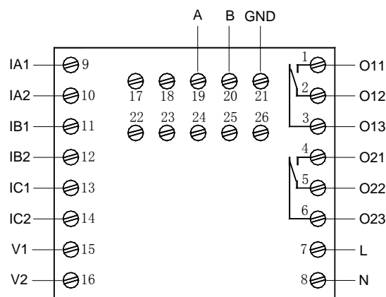
AMDP-□/□D242 系列保护器主单元接线端子图
