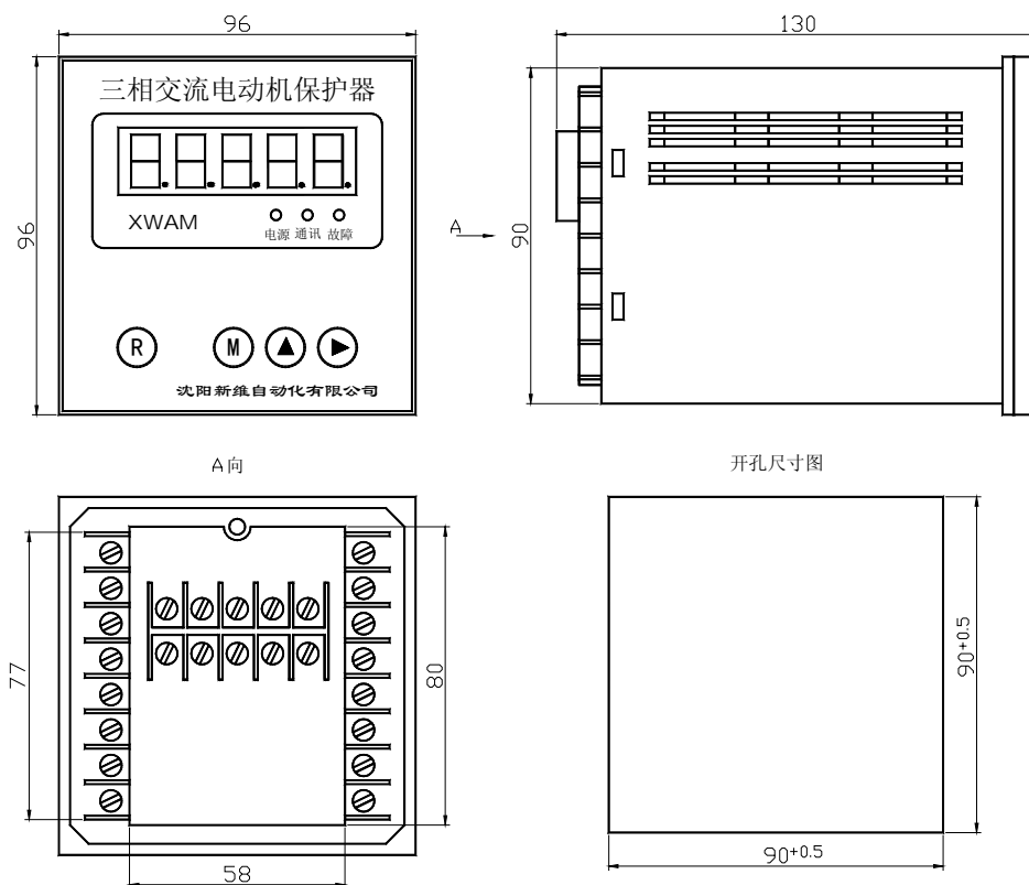
AMDP-□/24□ 系列电动机保护器主单元外形及安装孔尺寸
