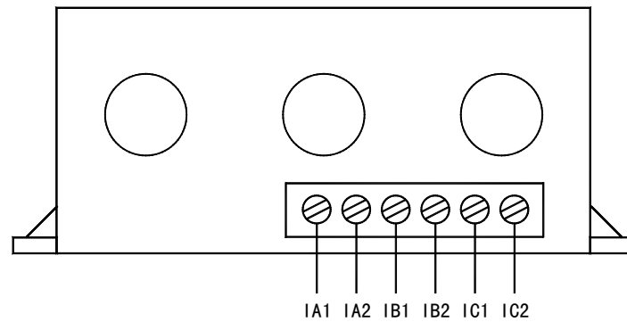
AMDP-□/□D24□ 系列保护器电流检测单元接线端子图
