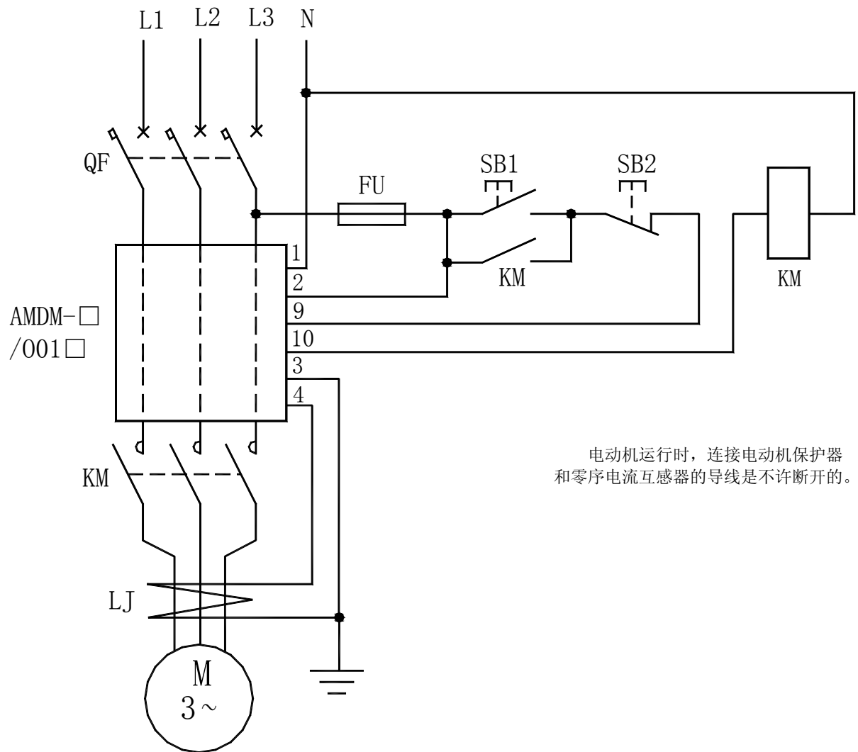
AMDM-□/001□ 系列电动机保护器应用电气原理图
