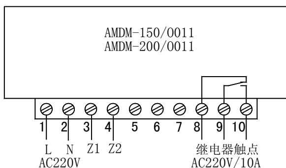
AMDM-□/0011 系列电动机保护器接线端子图
