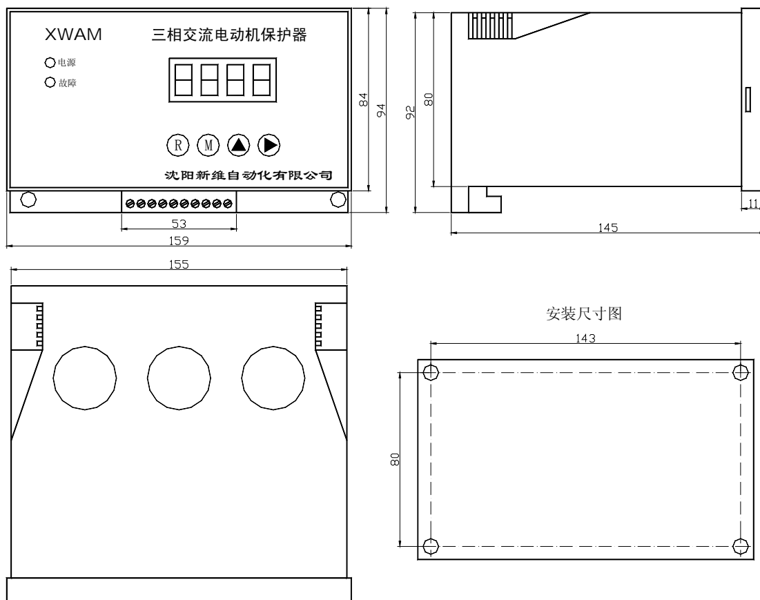
AMD-□/001□ 系统电动机保护器外形及安装孔尺寸
