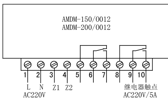
AMDM-□/0012 系列电动机保护器接线端子图
