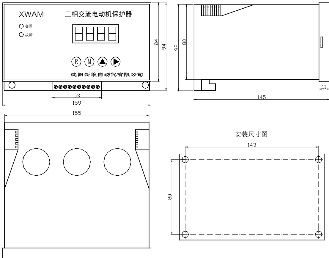
AMD-L-□/007□ 系统电动机保护器外形及安装孔尺寸
