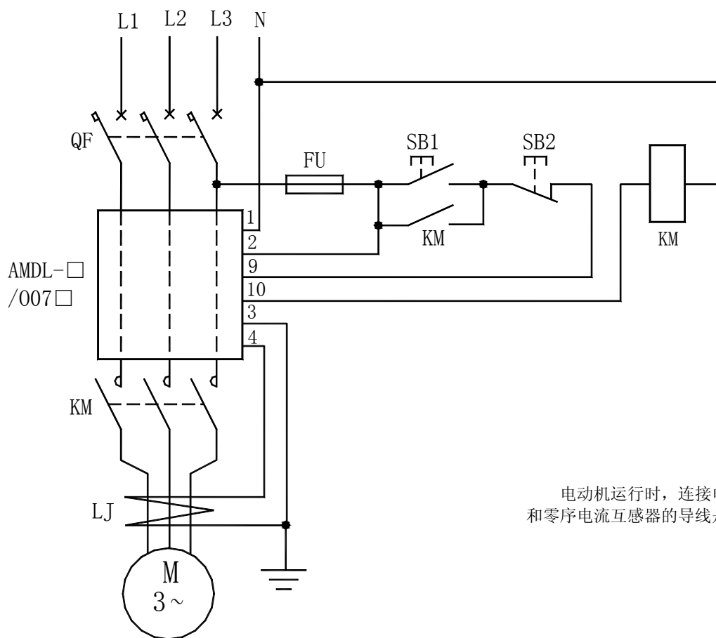
AMDL-□/007□ 系列电动机保护器应用电气原理图
