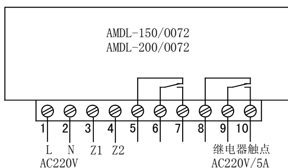
AMDL-□/0072 保护器接线端子图
