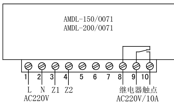
AMDL-□/0071 保护器接线端子图
