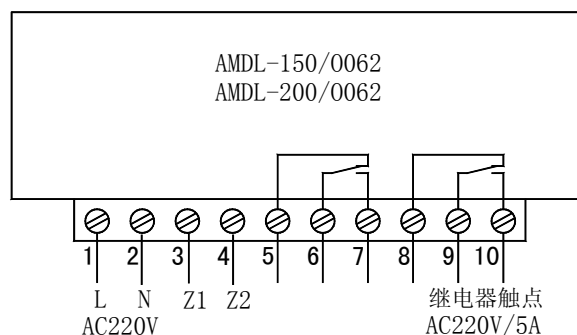
AMDL-□/0062 保护器接线端子图
