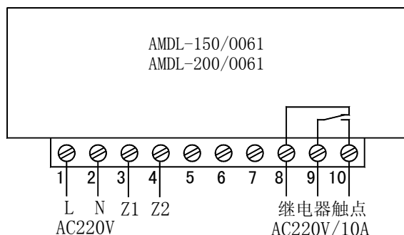
AMDL-□/0061 保护器接线端子图
