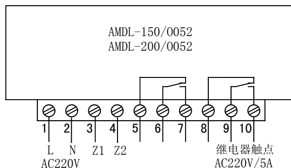
AMDL-□/0052 保护器接线端子图
