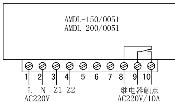
AMDL-□/0051 保护器接线端子图
