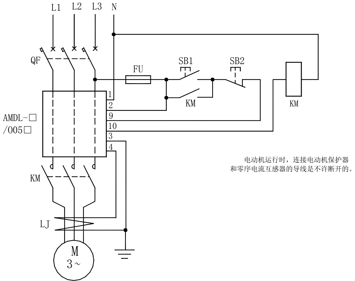
AMDL-□/005□ 系列电动机保护器应用电气原理图
