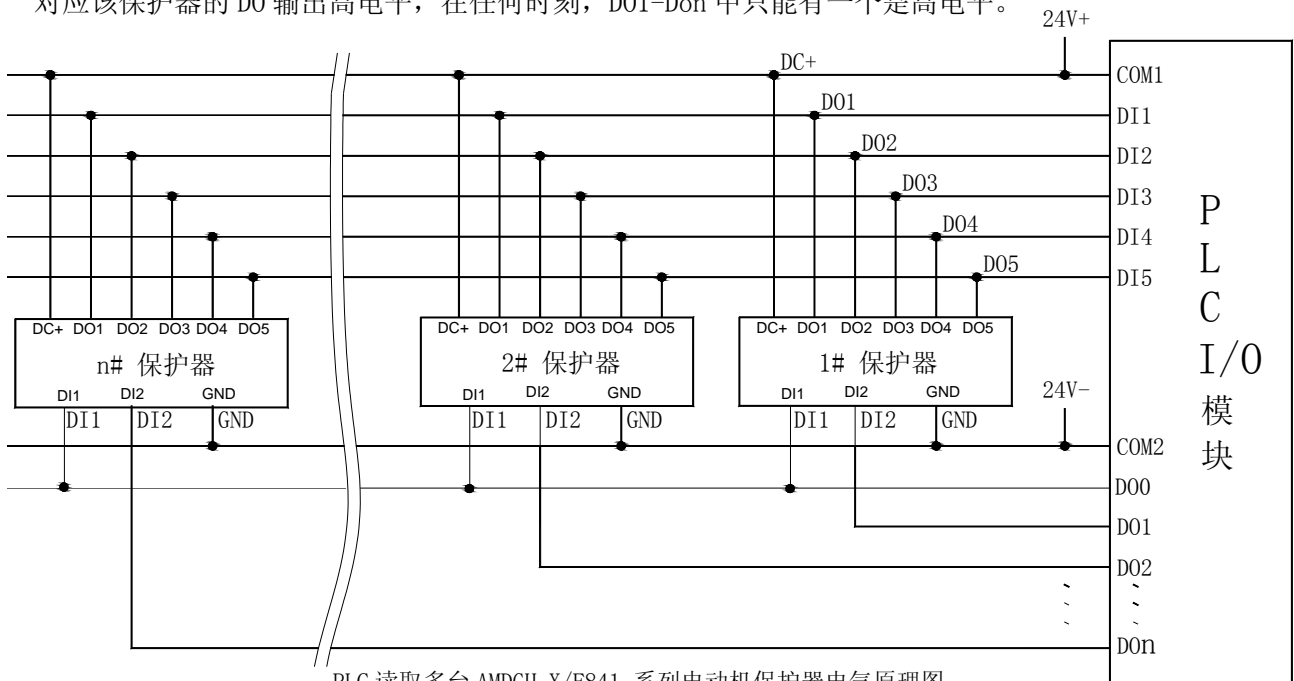
PLC 读取多台 AMDGH-X/F841 系列电动机保护器电气原理图
