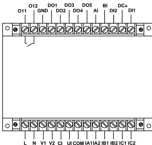
AMDGH-X/F841 系列保护器主单元接线端子图
