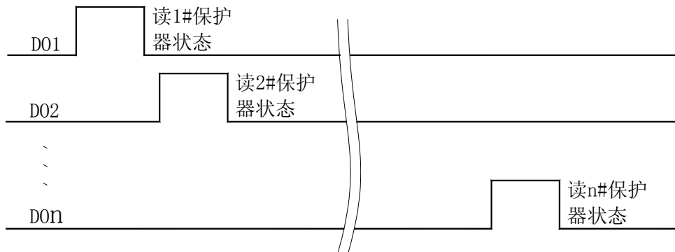
PLC 读取多台 AMDGH-X/F841 系列电动机保护器时序图
