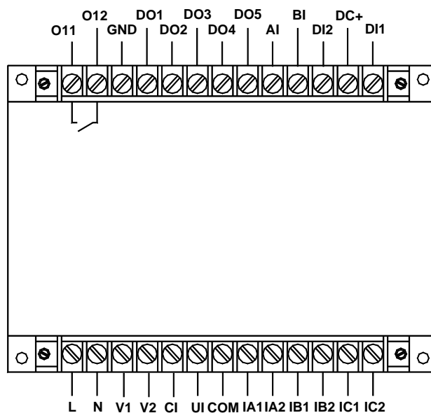
AMDGH-X/F821 系列保护器主单元接线端子图
