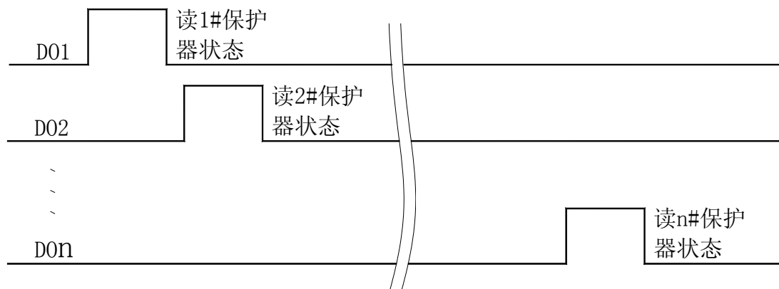
PLC 读取多台 AMDGH-X/F821 系列电动机保护器时序图
