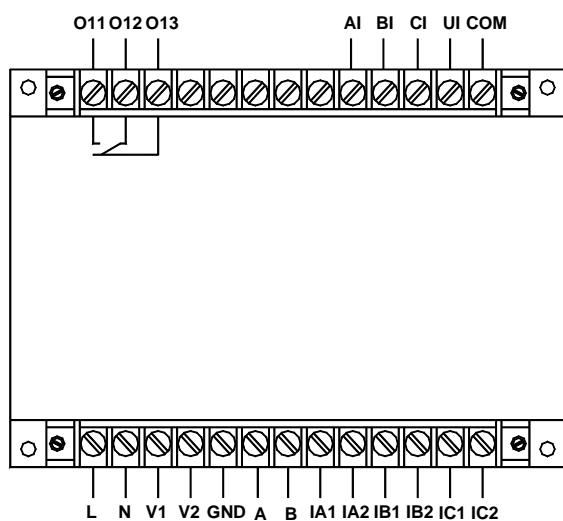
AMDGH-X/F421 系列保护器主单元接线端子图
