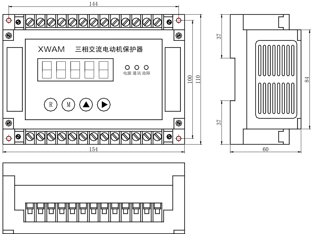
AMDGH-X/F42□ 系列电动机保护器主单元外形及安装孔尺寸
