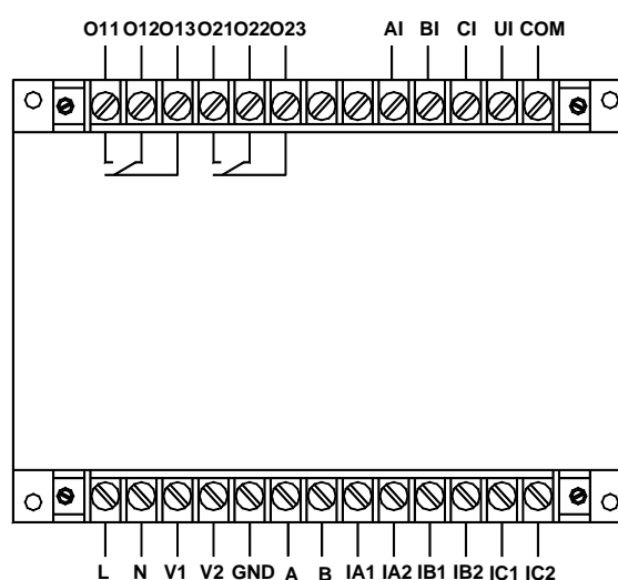
AMDGH-X/F422 系列保护器主单元接线端子图
