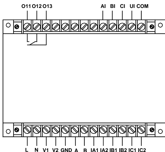
AMDGH-X/F401 系列保护器主单元接线端子图
