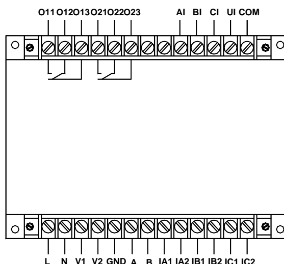
AMDGH-X/F402 系列保护器主单元接线端子图
