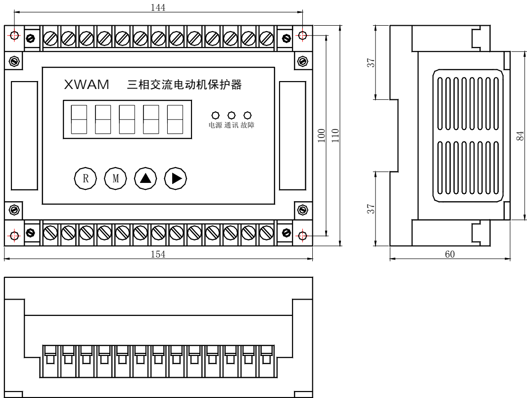
AMDGH-X/F40□ 系列电动机保护器主单元外形及安装孔尺寸
