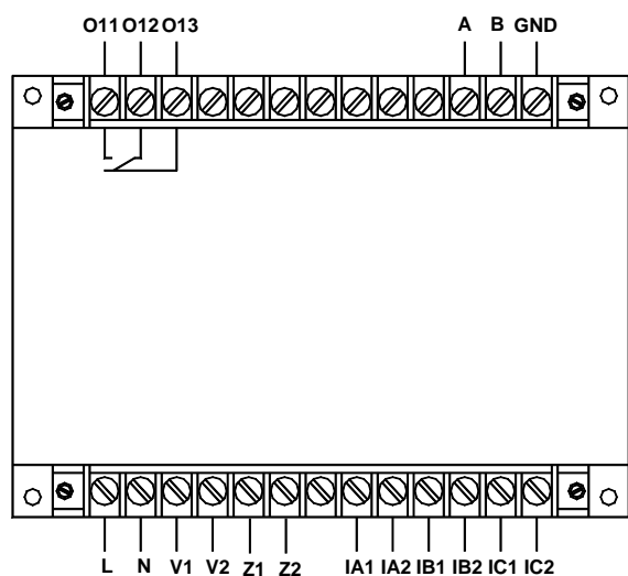
AMDGH-X/F371 系列保护器主单元接线端子图
