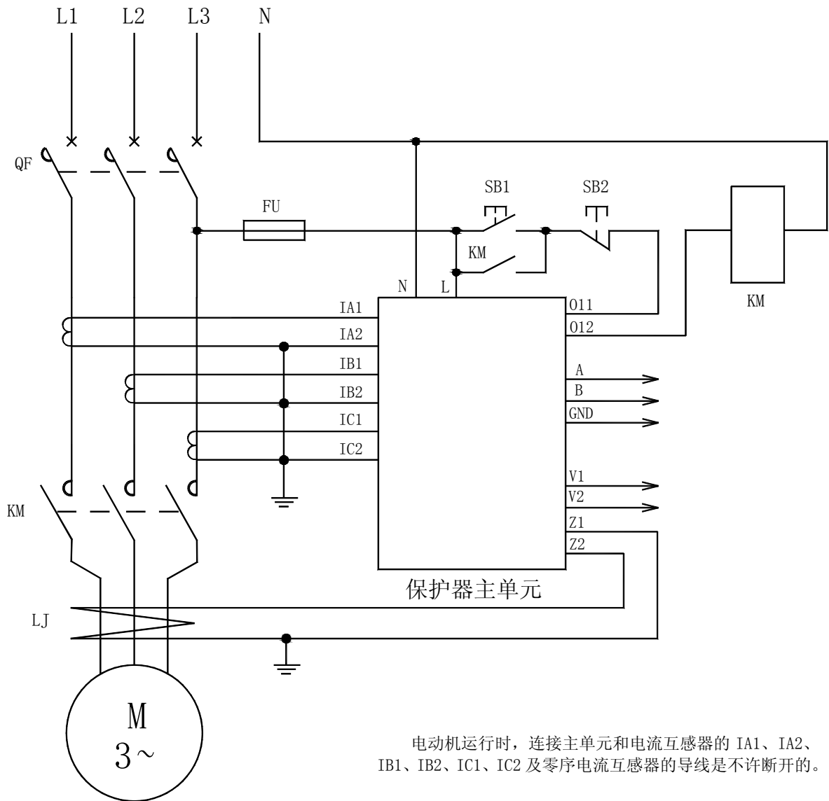
AMDGH-X/F37□ 系列电动机保护器应用电气原理图
