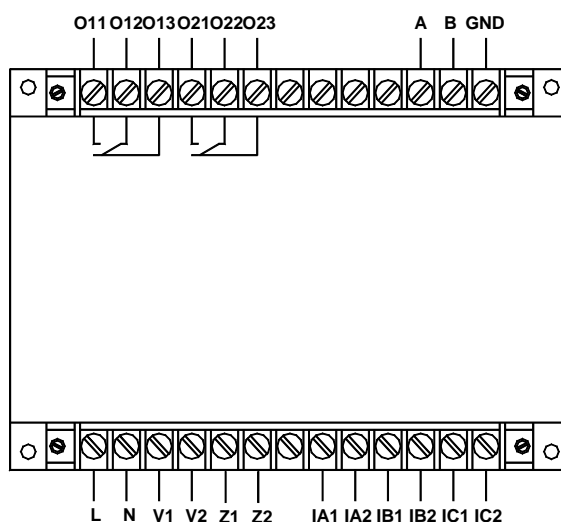
AMDGH-X/F372 系列保护器主单元接线端子图
