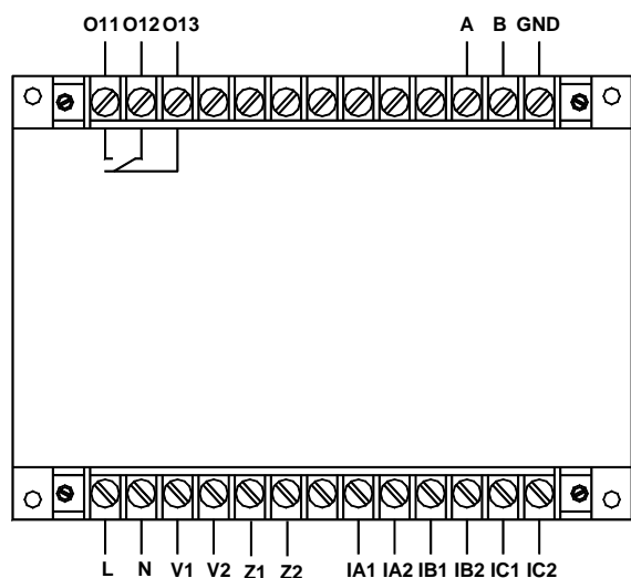
AMDGH-X/F361 系列保护器主单元接线端子图
