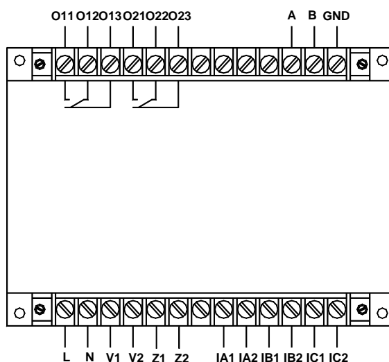
AMDGH-X/F362 系列保护器主单元接线端子图
