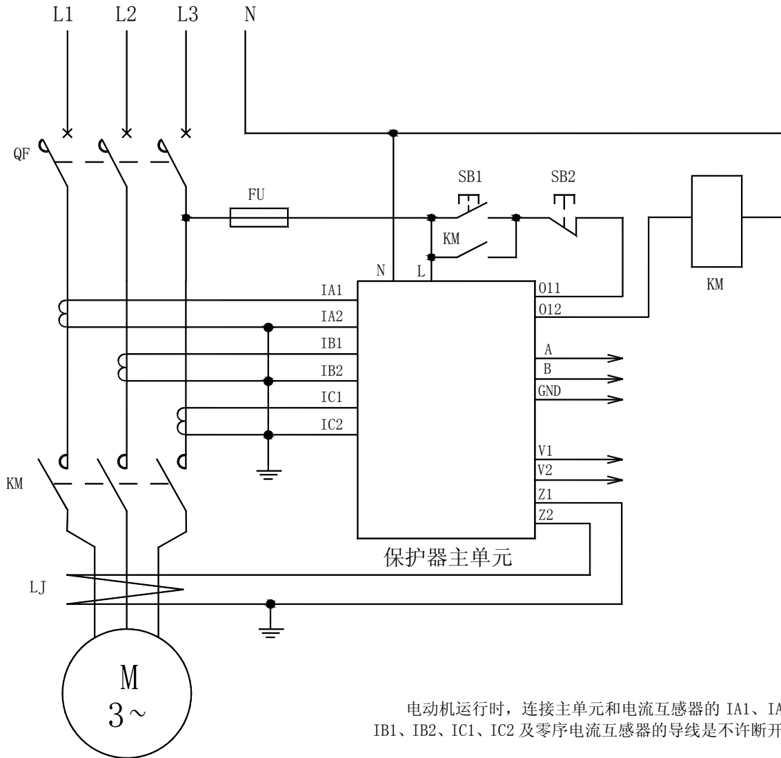
AMDGH-X/F36□ 系列电动机保护器应用电气原理图
