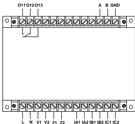
AMDGH-X/F351 系列保护器主单元接线端子图
