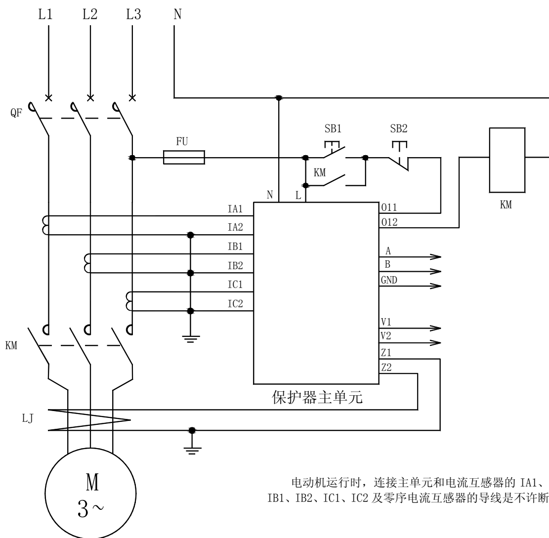
AMDGH-X/F35□ 系列电动机保护器应用电气原理图
