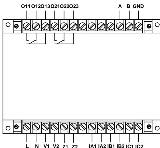
AMDGH-X/F352 系列保护器主单元接线端子图
