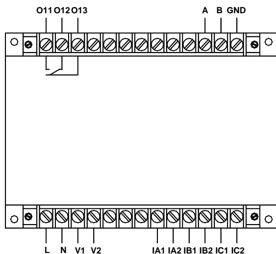
AMDGH-X/F341 系列保护器主单元接线端子图 沈阳新维自动化有限公司
