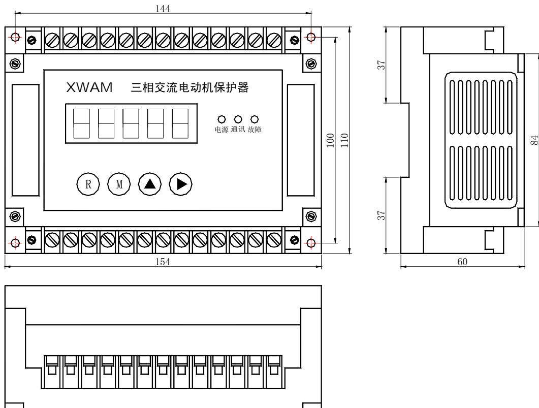
AMDGH-X/F34□ 系列电动机保护器主单元外形及安装孔尺寸
