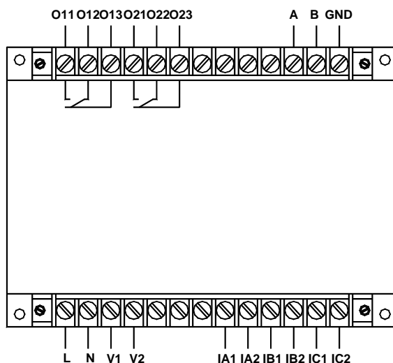
AMDGH-X/F342 系列保护器主单元接线端子图 HTTP://WWW.SY-XINWEI.COM
