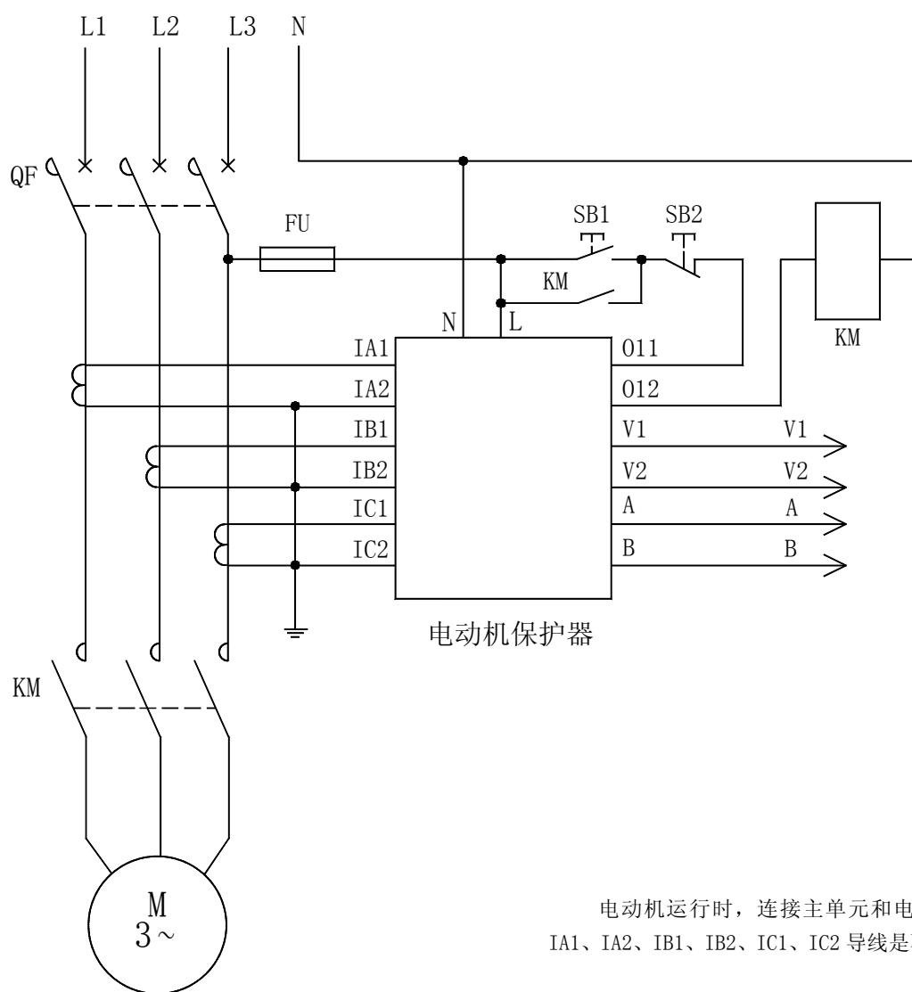
AMDGH-X/F33□ 系列电动机保护器应用电气原理图
