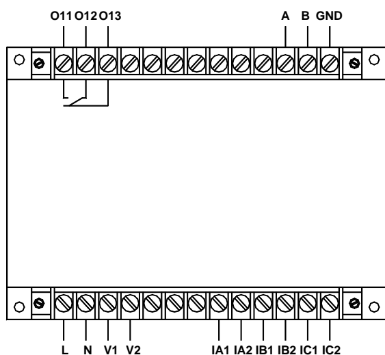
AMDGH-X/F331 系列保护器主单元接线端子图
