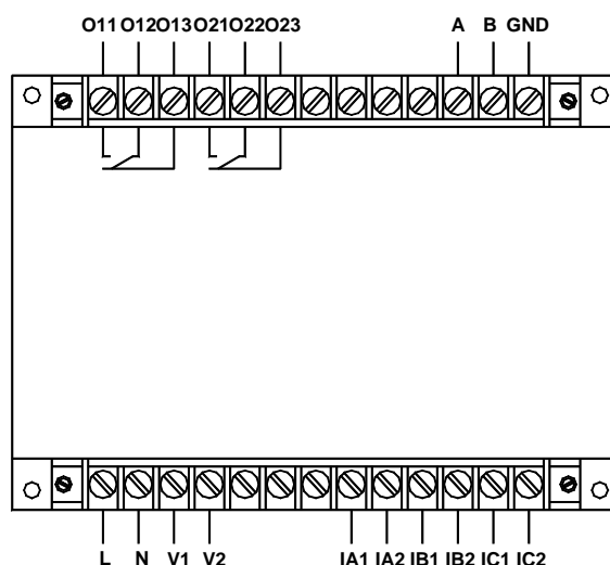
AMDGH-X/F332 系列保护器主单元接线端子图
