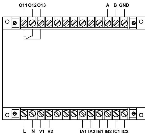
AMDGH-X/F321 系列保护器主单元接线端子图
