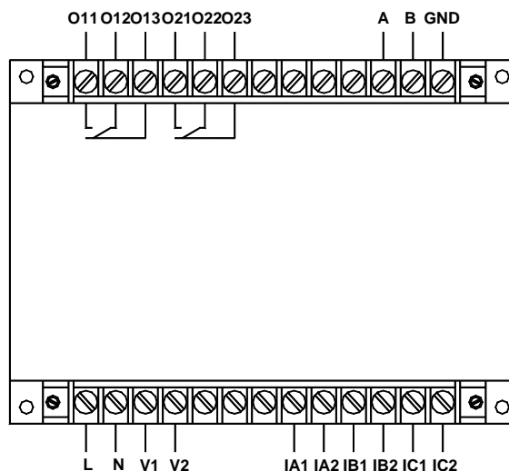
AMDGH-X/F322 系列保护器主单元接线端子图
