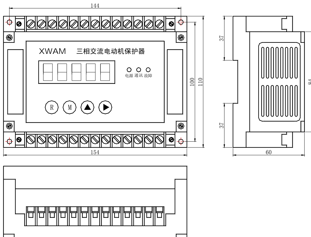
AMDGH-X/F32□ 系列电动机保护器主单元外形及安装孔尺寸
