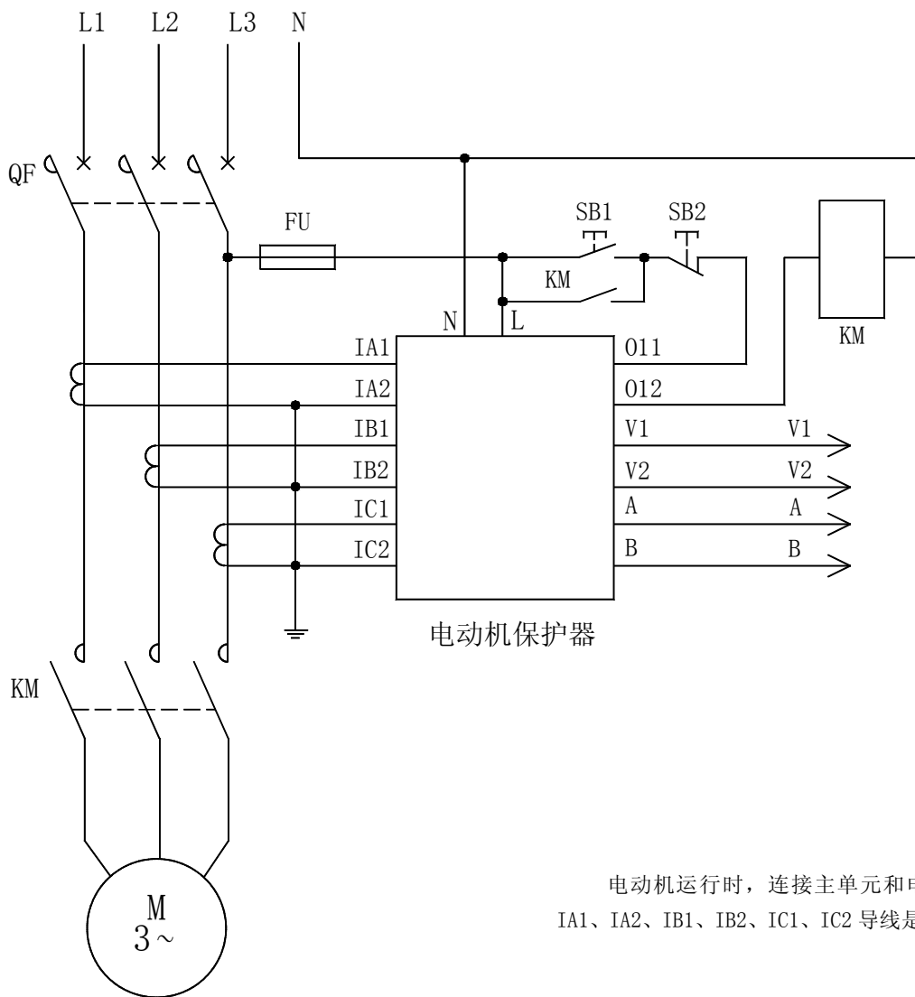
AMDGH-X/F32□ 系列电动机保护器应用电气原理图
