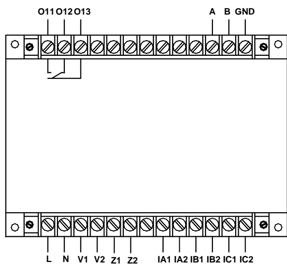
AMDGH-X/F311 系列保护器主单元接线端子图
