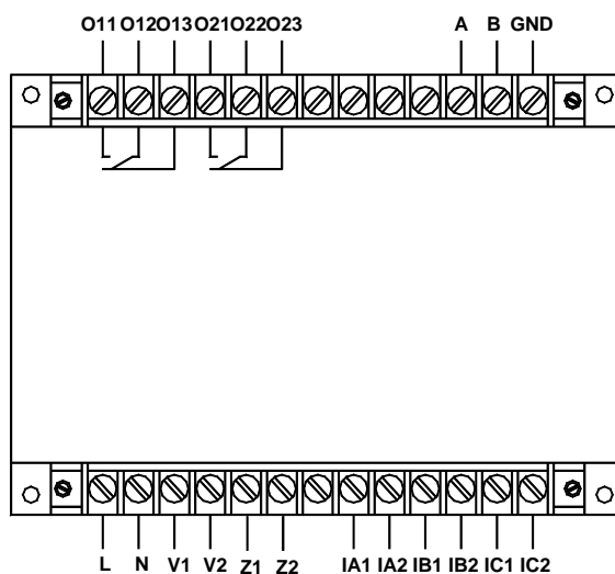
AMDGH-X/F312 系列保护器主单元接线端子图
