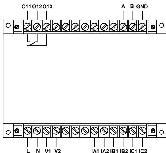
AMDGH-X/F301 系列保护器主单元接线端子图
