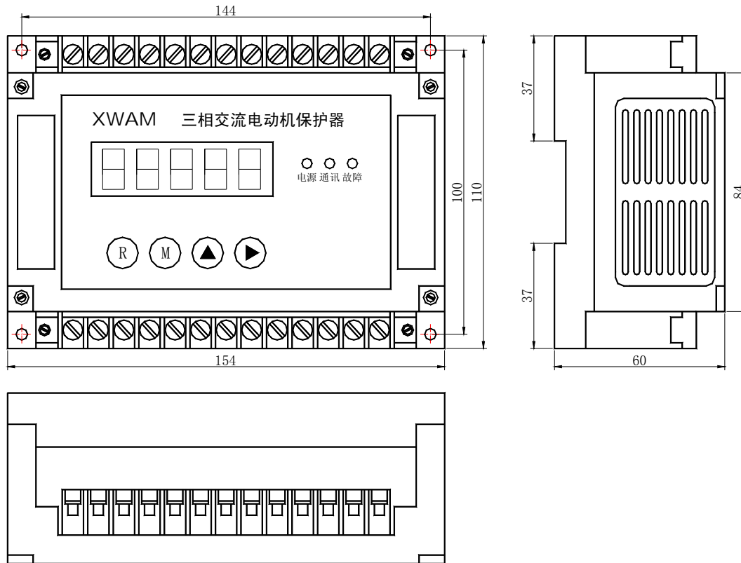
AMDGH-X/F30□ 系列电动机保护器主单元外形及安装孔尺寸
