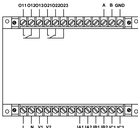
AMDGH-X/F302 系列保护器主单元接线端子图
