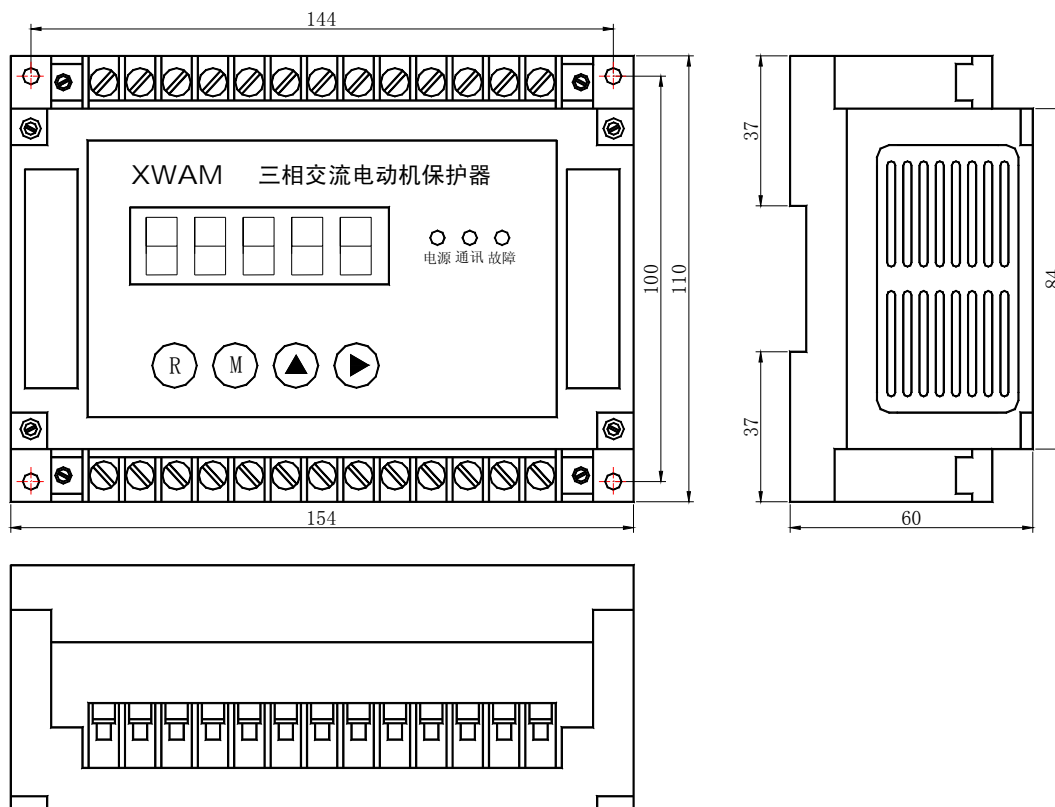
AMDGH-X/F26□ 系列电动机保护器主单元外形及安装孔尺寸
