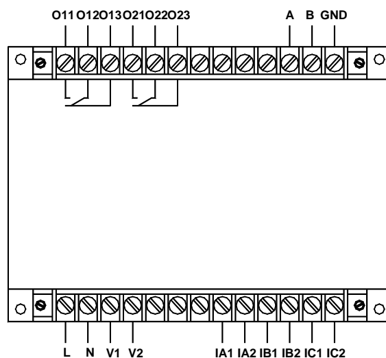
AMDGH-X/F232 系列保护器主单元接线端子图
