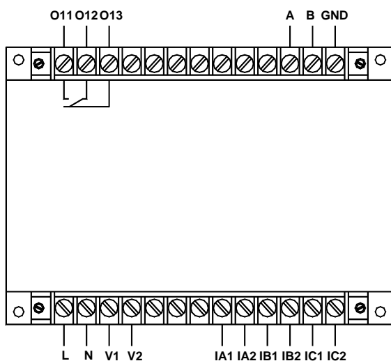
AMDGH-X/F231 系列保护器主单元接线端子图
