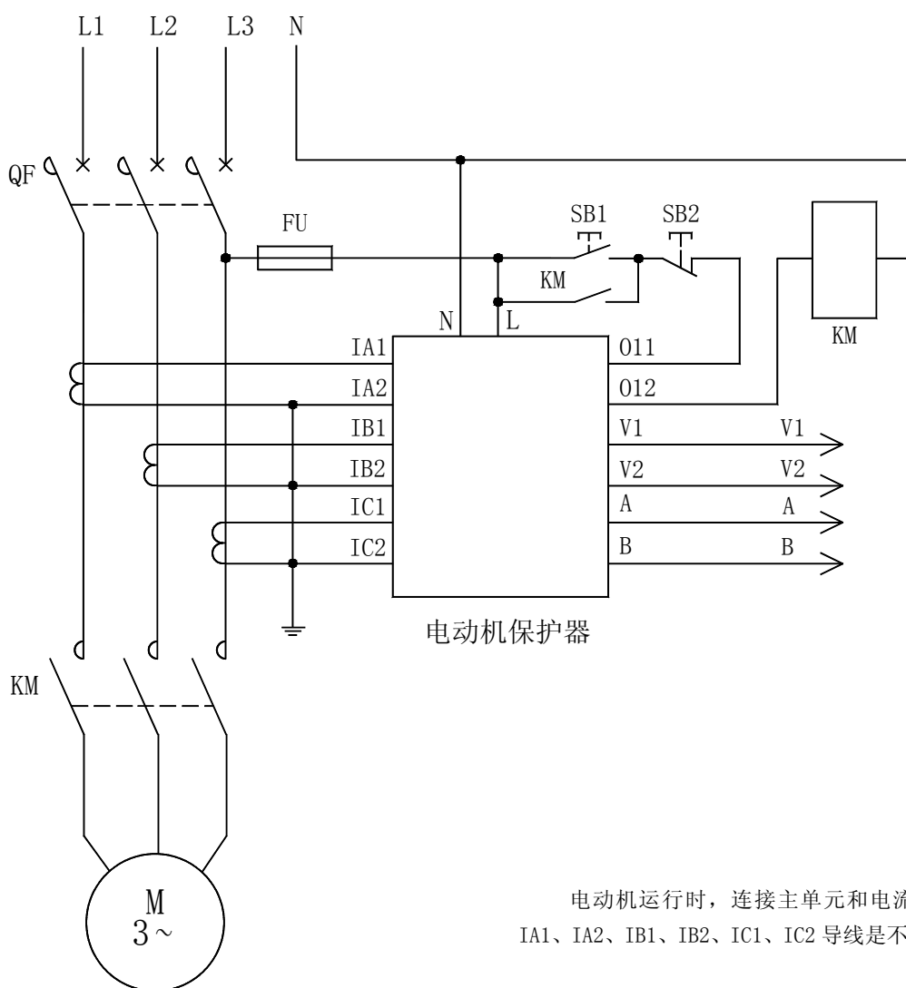
AMDGH-X/F23□ 系列电动机保护器应用电气原理图
