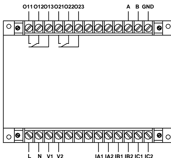
AMDGH-X/F222 系列保护器主单元接线端子图
