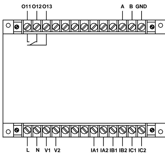
AMDGH-X/F221 系列保护器主单元接线端子图
