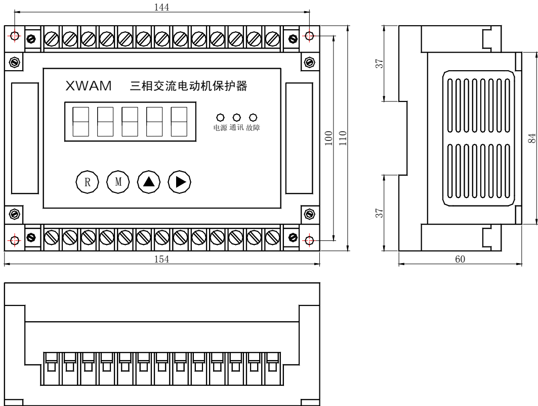
AMDGH-X/F21□ 系列电动机保护器主单元外形及安装孔尺寸
