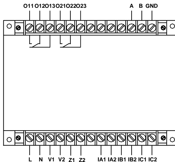
AMDGH-X/F212 系列保护器主单元接线端子图
