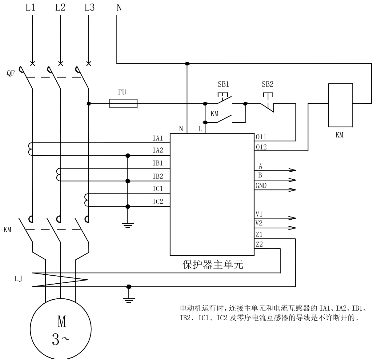
AMDGH-X/F21 □ 系列电动机保护器应用电气原理图
