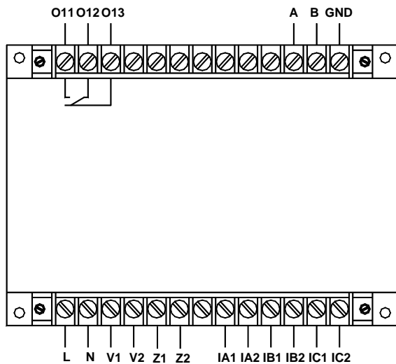
AMDGH-X/F211 系列保护器主单元接线端子图
