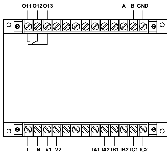
AMDGH-X/F201 系列保护器主单元接线端子图
