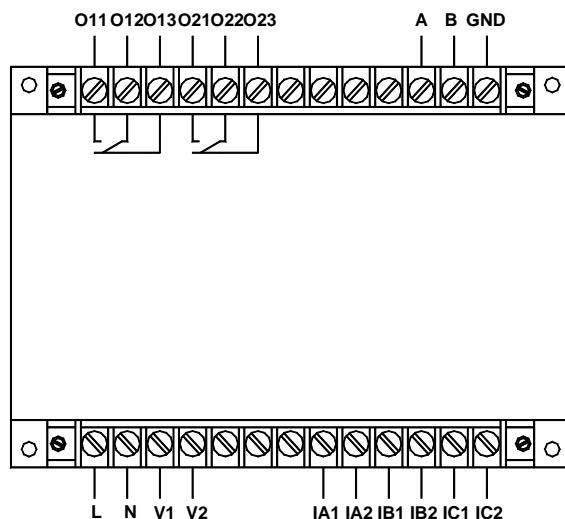
AMDGH-X/F202 系列保护器主单元接线端子图
