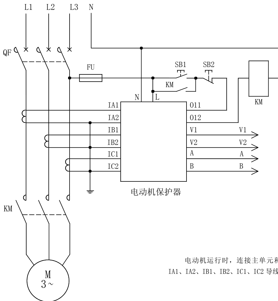
AMDGH-X/F20 系列电动机保护器应用电气原理图
