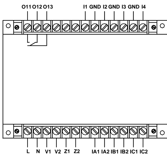
AMDGH-X/F171 系列保护器主单元接线端子图
