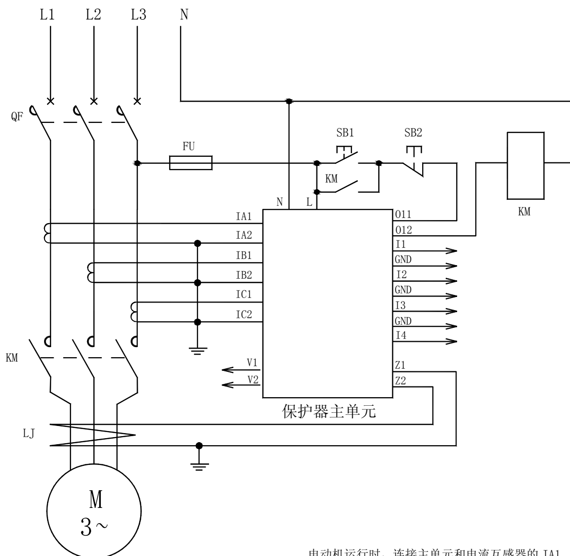
AMDGH-X/F17□ 系列电动机保护器应用电气原理图
