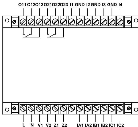
AMDGH-X/F172 系列保护器主单元接线端子图
