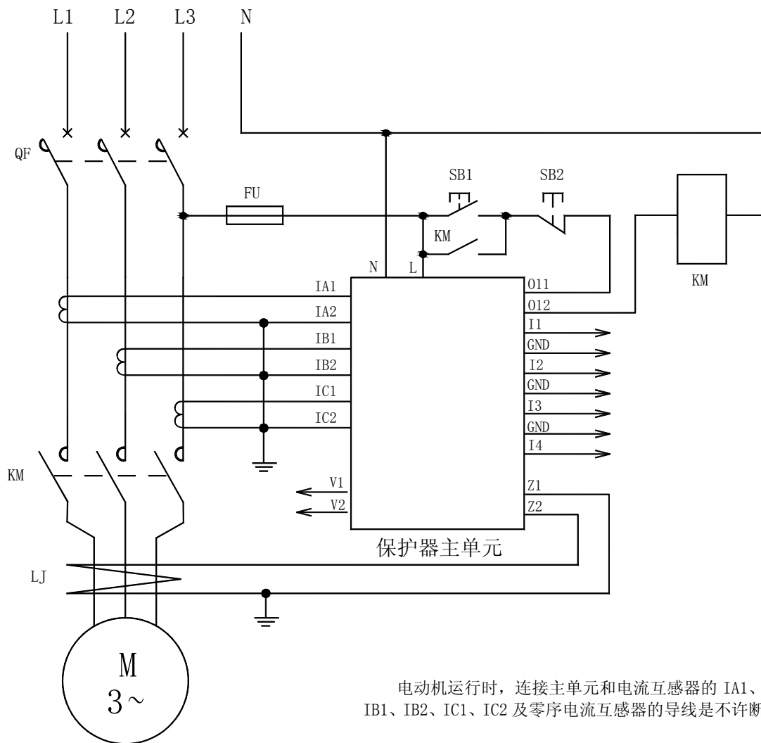
AMDGH-X/F16□ 系列电动机保护器应用电气原理图
