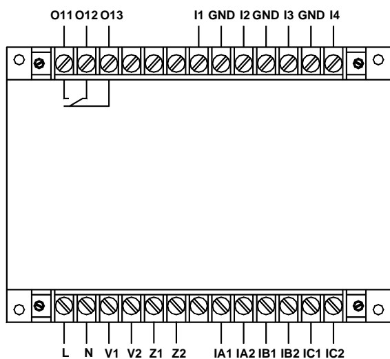
AMDGH-X/F161 系列保护器主单元接线端子图
