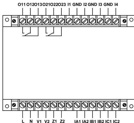
AMDGH-X/F162 系列保护器主单元接线端子图
