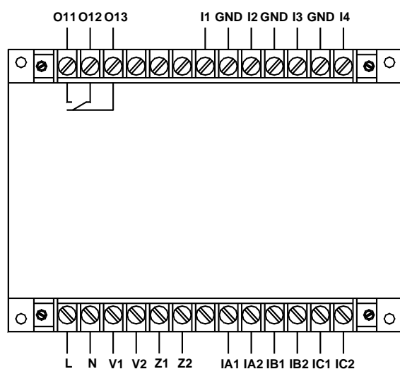
AMDGH-X/F151 系列保护器主单元接线端子图
