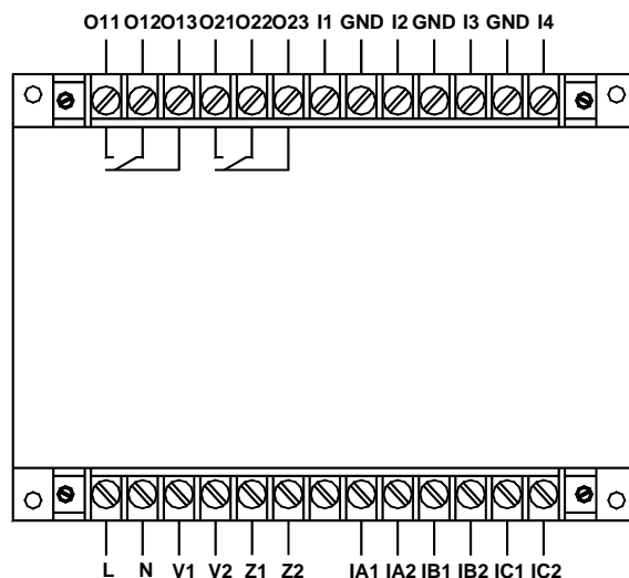
AMDGH-X/F152 系列保护器主单元接线端子图
