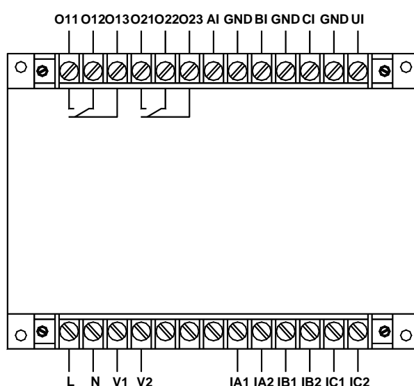
AMDGH-X/F142 系列保护器主单元接线端子图
