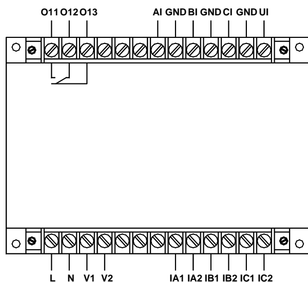
AMDGH-X/F141 系列保护器主单元接线端子图
