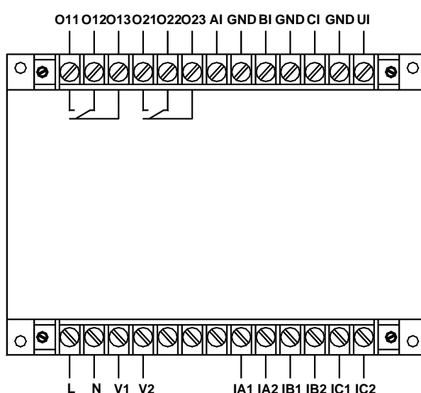
AMDGH-X/F132 系列保护器主单元接线端子图
