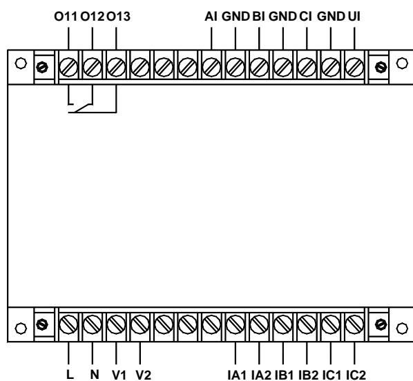
AMDGH-X/F131 系列保护器主单元接线端子图
