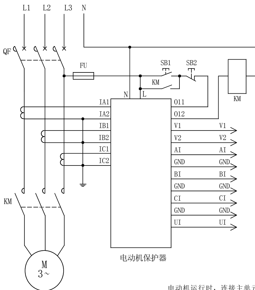
AMDGH-X/F13□ 系列电动机保护器应用电气原理图
