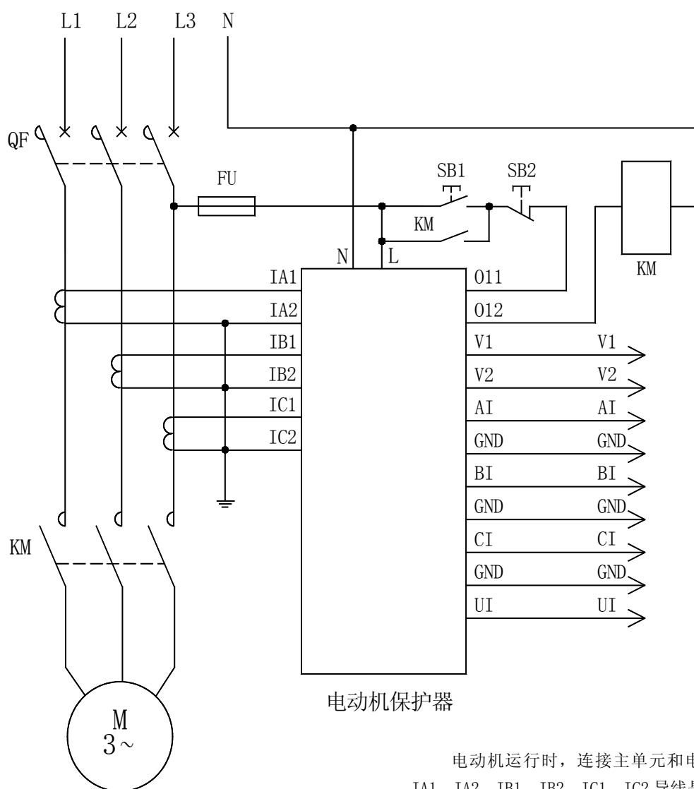
AMDGH-X/F12□ 系列电动机保护器应用电气原理图
