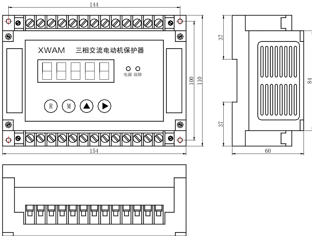
AMDGH-X/F12□ 系列电动机保护器主单元外形及安装孔尺寸
