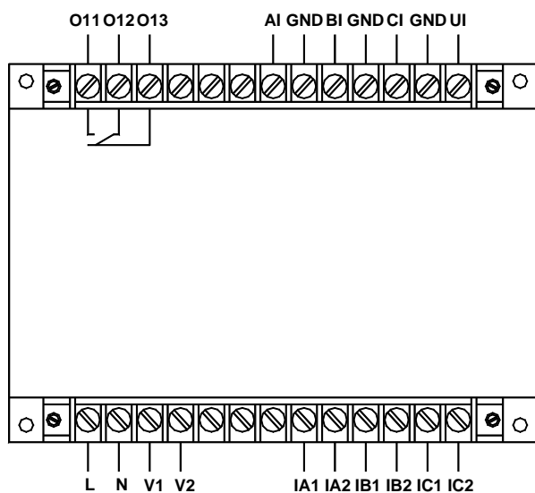
AMDGH-X/F121 系列保护器主单元接线端子图
