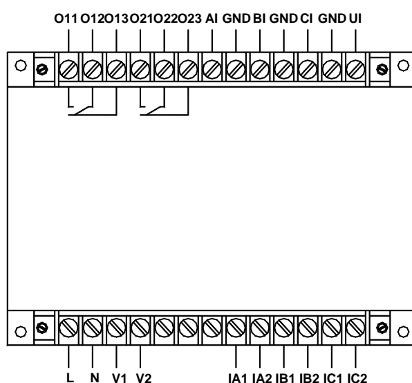
AMDGH-X/F122 系列保护器主单元接线端子图
