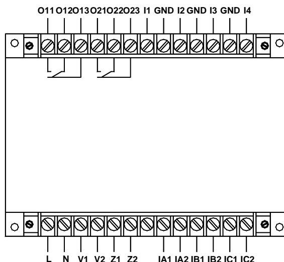
AMDGH-X/F112 系列保护器主单元接线端子图
