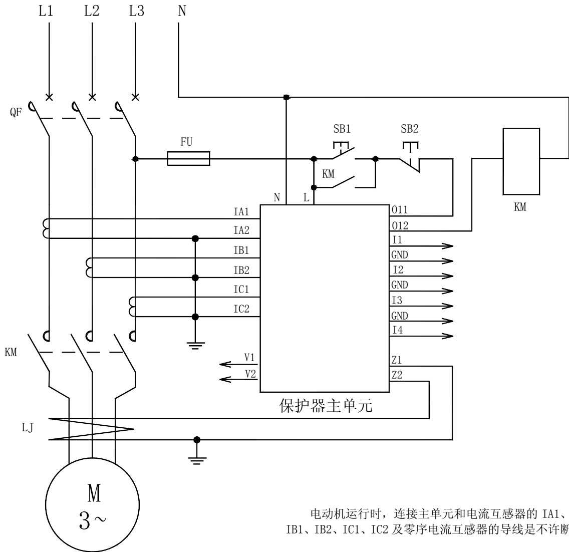
AMDGH-X/F11□ 系列电动机保护器应用电气原理图
