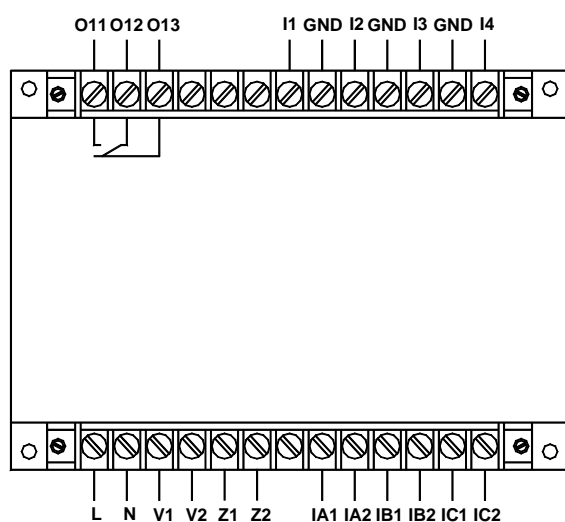
AMDGH-X/F111 系列保护器主单元接线端子图
