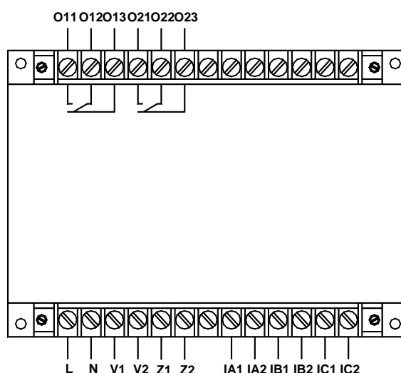
AMDGH-X/F072 系列保护器主单元接线端子图
