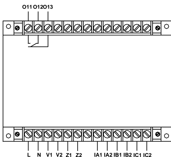
AMDGH-X/F071 系列保护器主单元接线端子图
