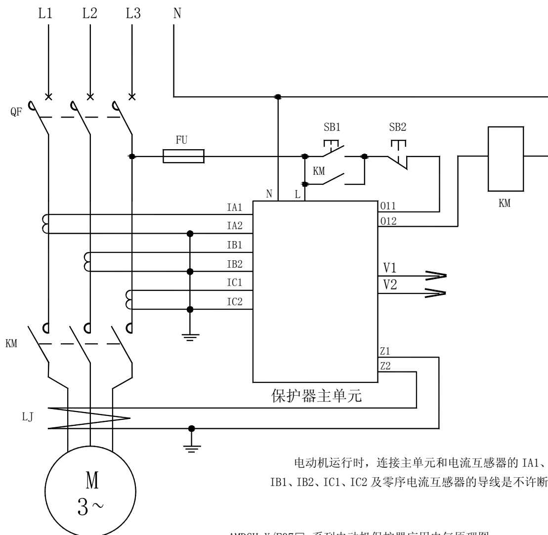
AMDGH-X/F07□ 系列电动机保护器应用电气原理图
