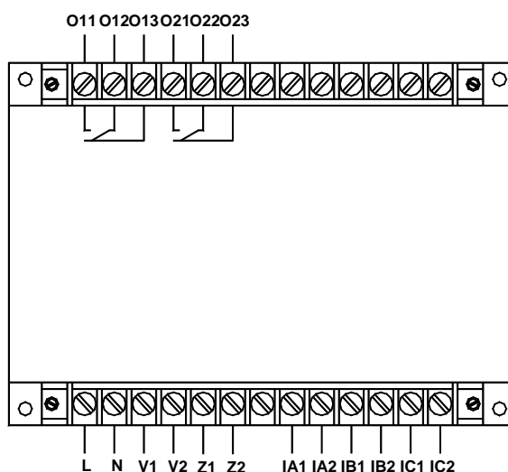
AMDGH-X/F062 系列保护器主单元接线端子图
