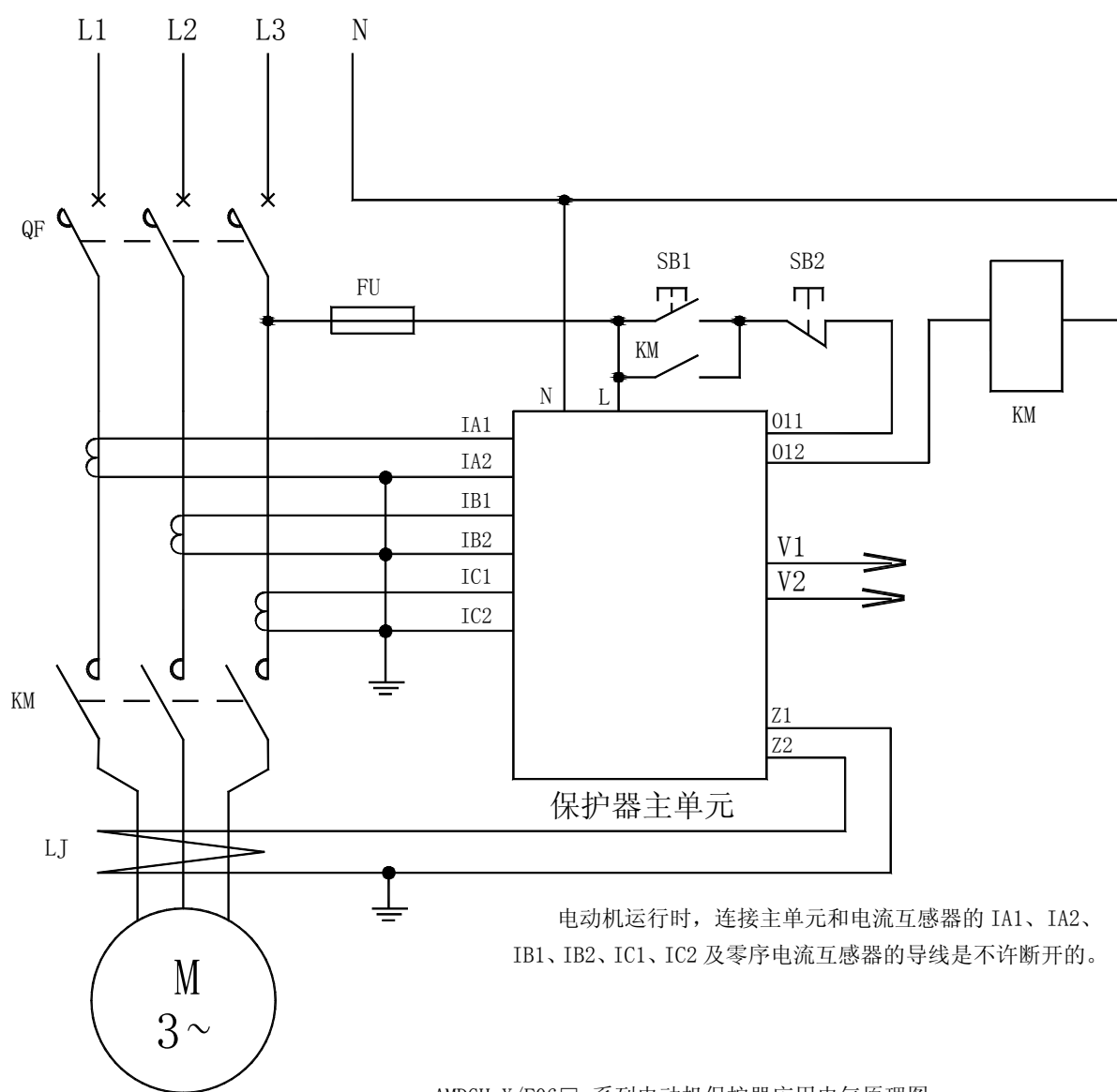
AMDGH-X/F06□ 系列电动机保护器应用电气原理图
