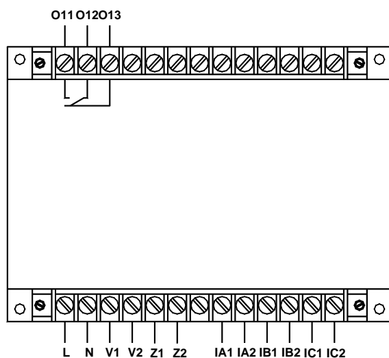
AMDGH-X/F061 系列保护器主单元接线端子图
