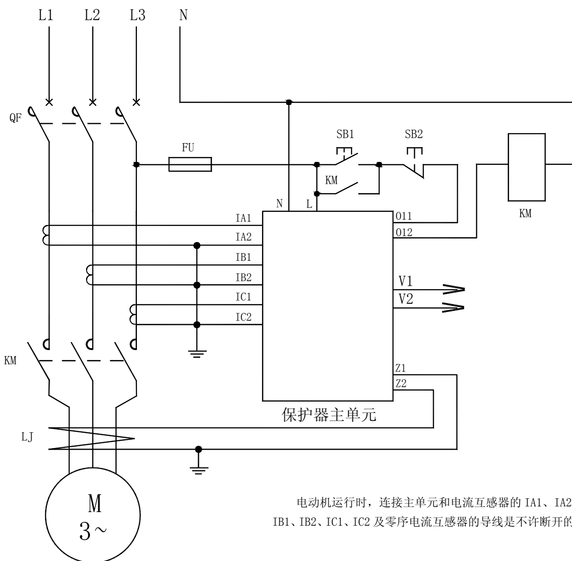
AMDGH-X/F05□ 系列电动机保护器应用电气原理图
