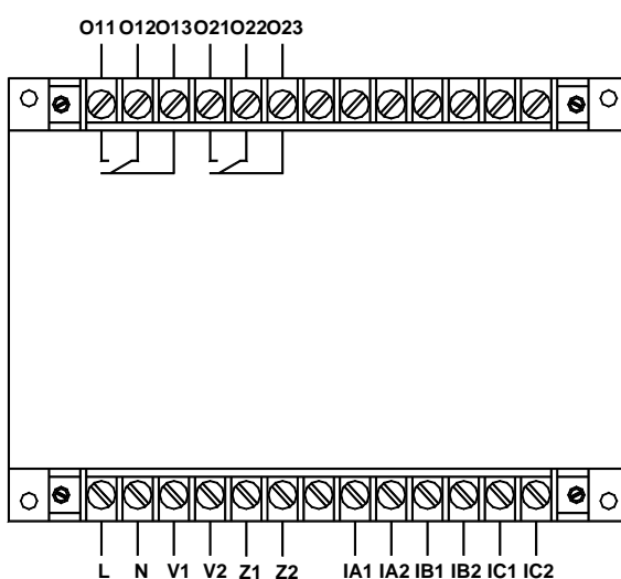
AMDGH-X/F052 系列保护器主单元接线端子图
