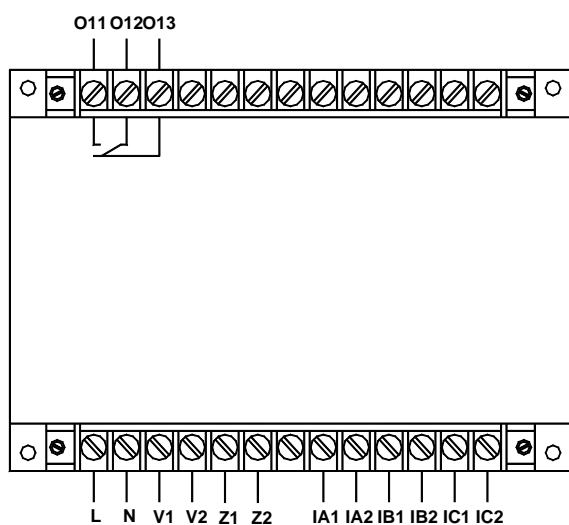
AMDGH-X/F051 系列保护器主单元接线端子图
