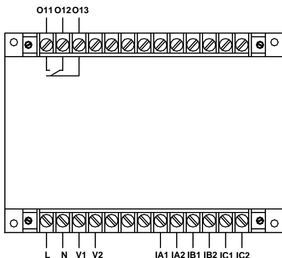
AMDGH-X/F031 系列保护器主单元接线端子图
