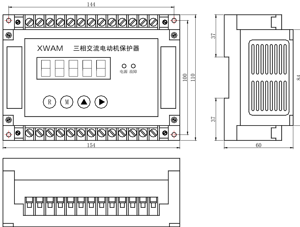
AMDGH-X/F03□ 系列电动机保护器主单元外形及安装孔尺寸
