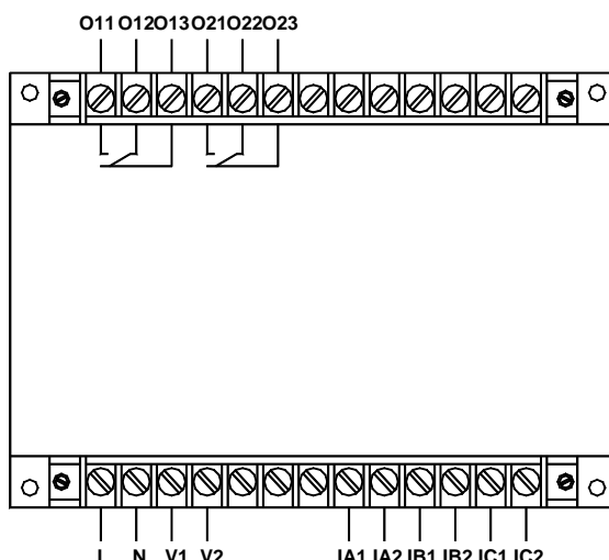
AMDGH-X/F032 系列保护器主单元接线端子图
