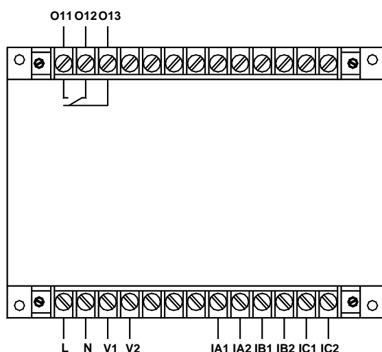
AMDGH-X/F021 系列保护器主单元接线端子图
