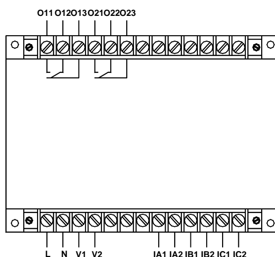
AMDGH-X/F022 系列保护器主单元接线端子图
