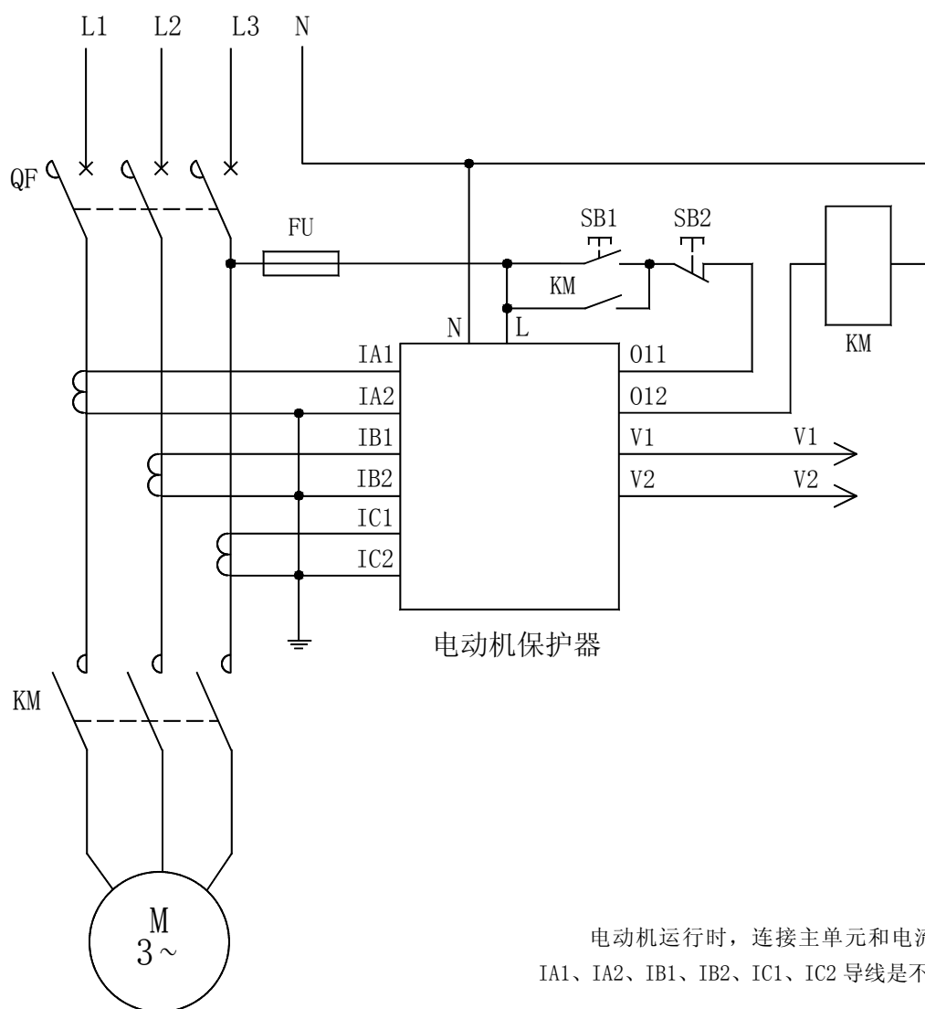
AMDGH-X/F02□ 系列电动机保护器应用电气原理图
