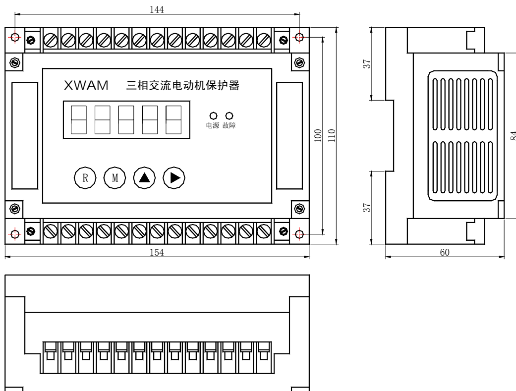
AMDGH-X/F02□ 系列电动机保护器主单元外形及安装孔尺寸
