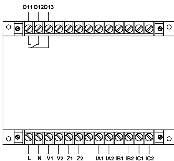
AMDGH-X/F011 系列保护器主单元接线端子图
