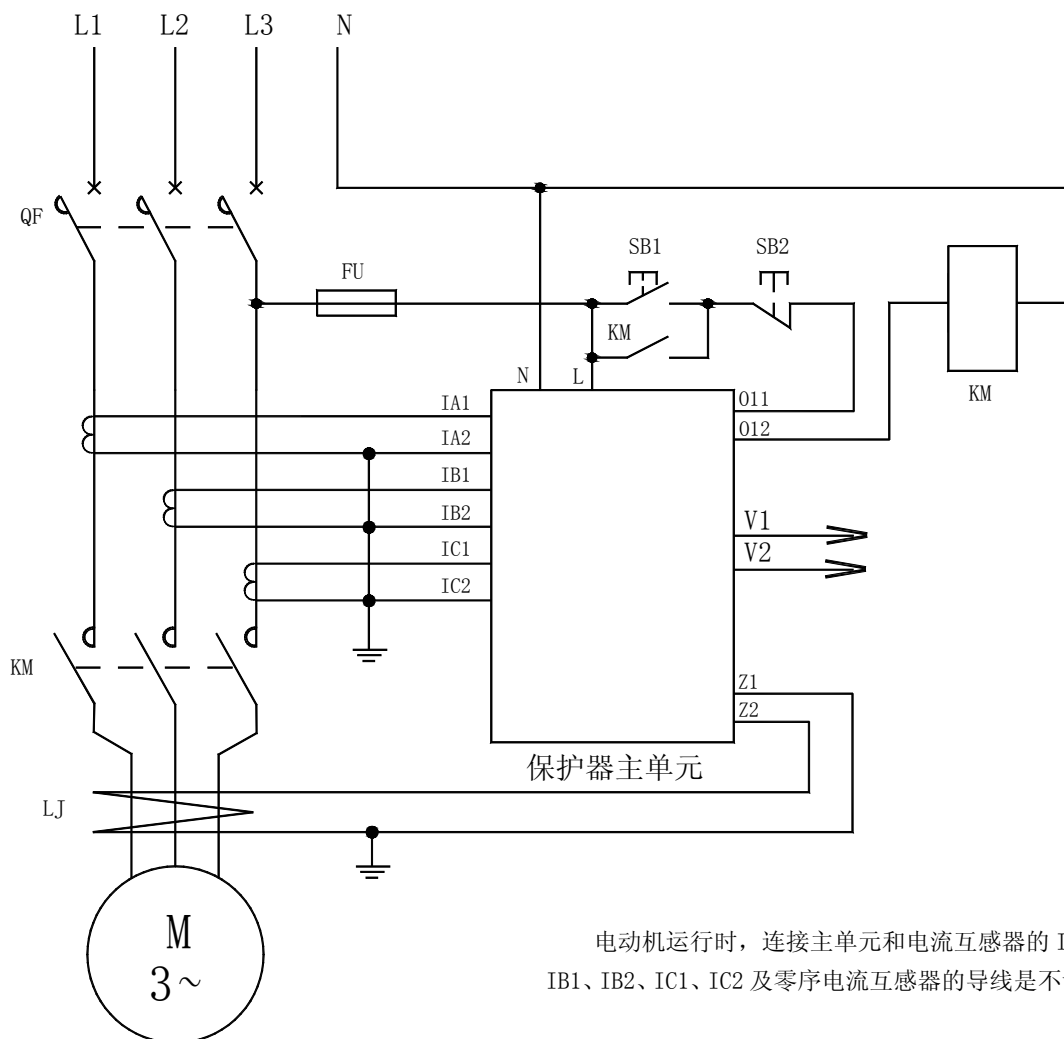
AMDGH-X/F01□ 系列电动机保护器应用电气原理图
