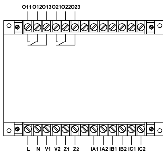
AMDGH-X/F012 系列保护器主单元接线端子图
