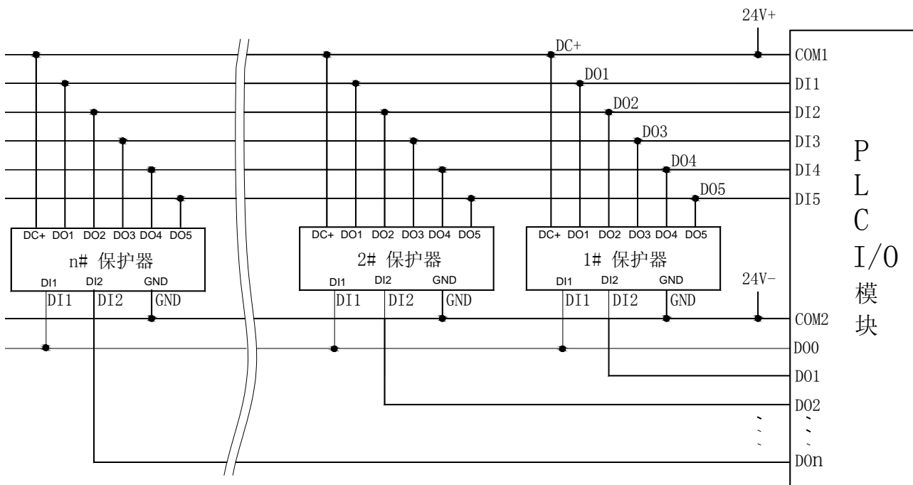
PLC 读取多台 AMDGH-X/E611 系列电动机保护器电气原理图
