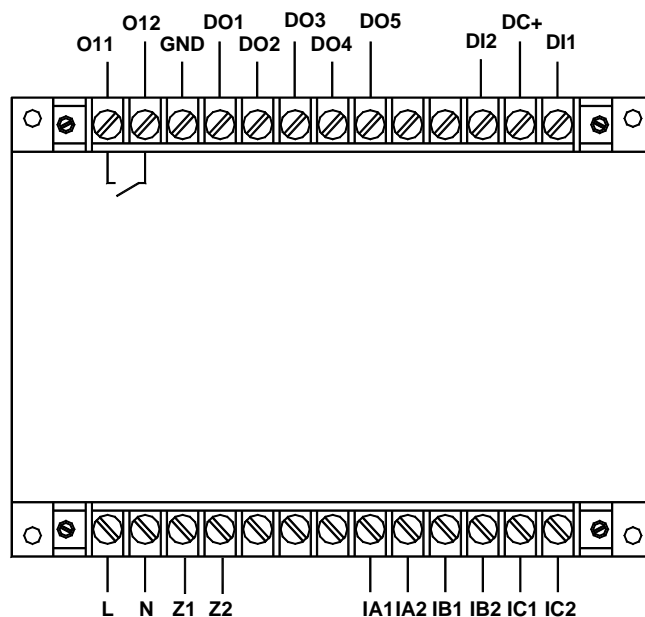
AMDGH-X/E611 系列保护器主单元接线端子图
