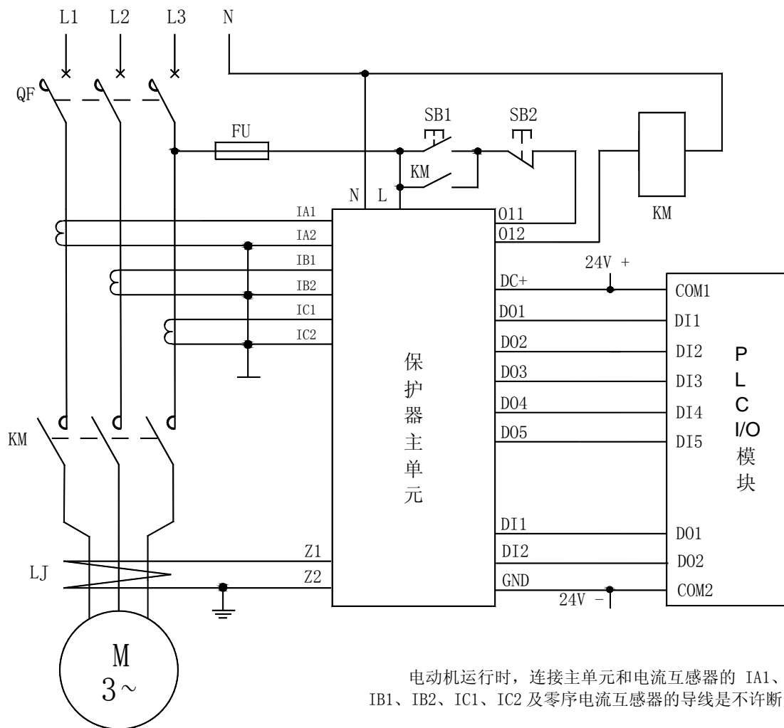
AMDGH-X/E611 系列电动机保护器 D0 连接 PLC 电气原理图
