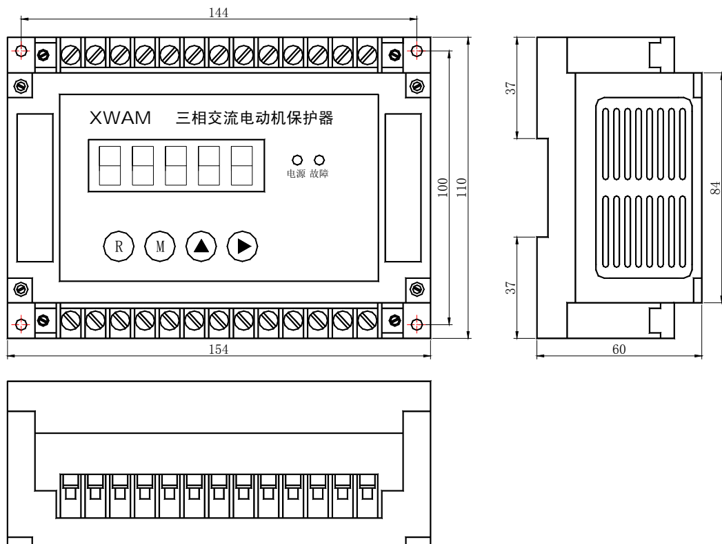
AMDGH-X/E611 系列电动机保护器主单元外形及安装孔尺寸
