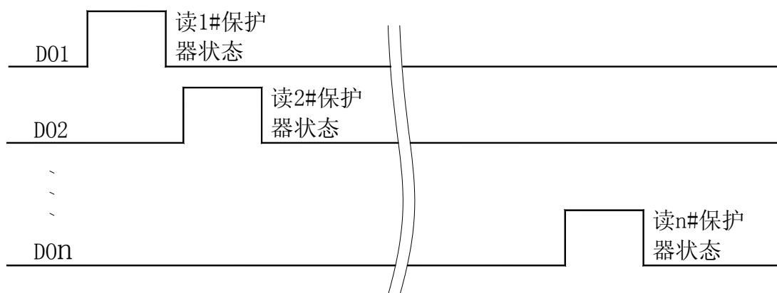
PLC 读取多台 AMDGH-X/E611 系列电动机保护器时序图
