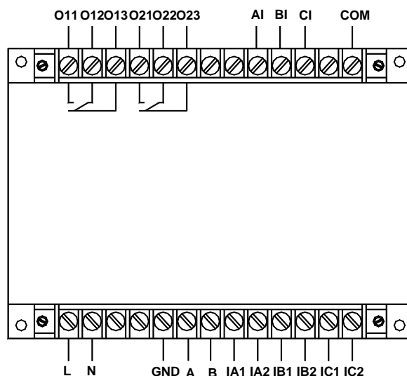
AMDG-X/E402 系列保护器主单元接线端子图
