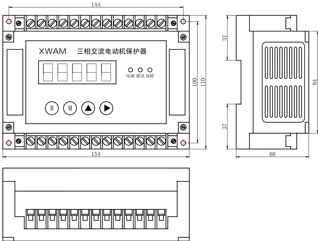
AMDG-X/E40□ 系列电动机保护器主单元外形及安装孔尺寸
