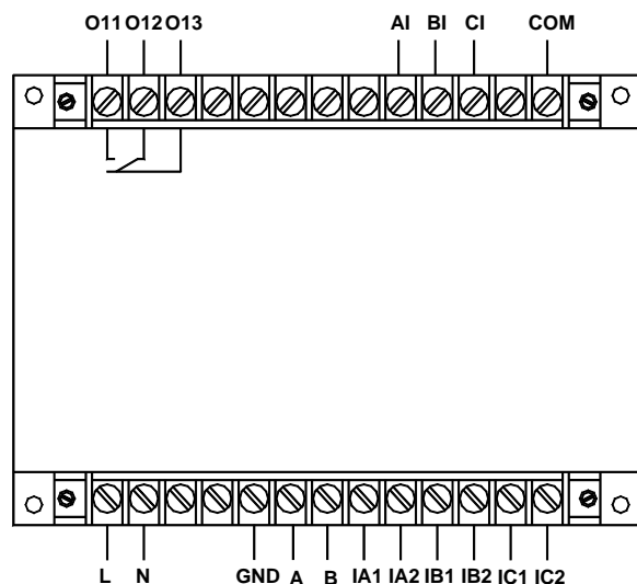
AMDG-X/E401 系列保护器主单元接线端子图
